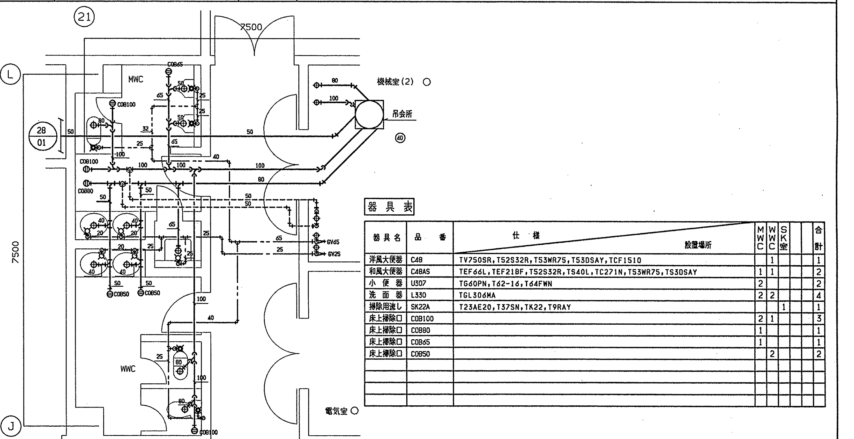
03 1階WC(2)平面詳細図 1/50
