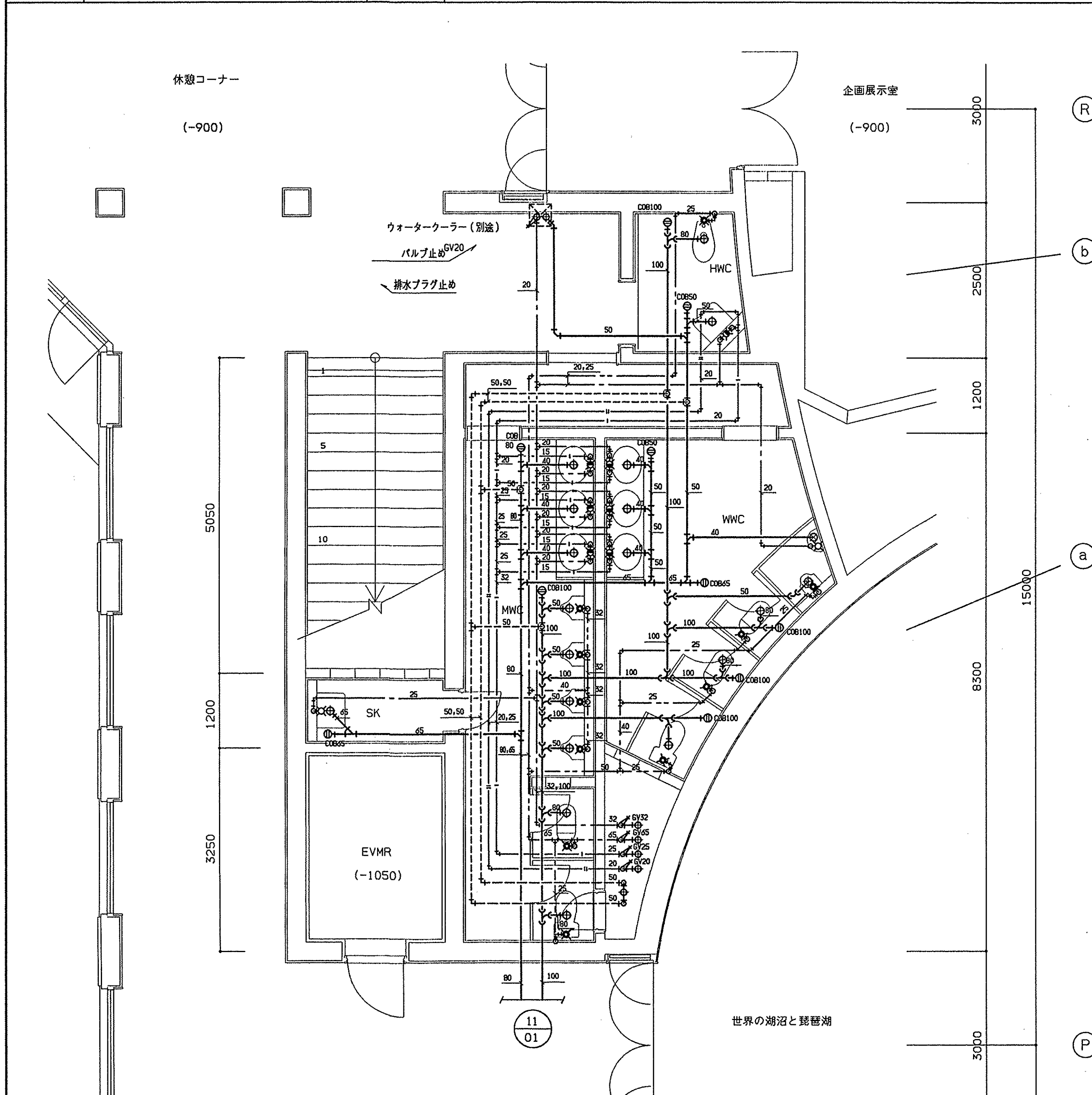
01 1階客用WC ( 4 ) 平面詳細図 1/50
