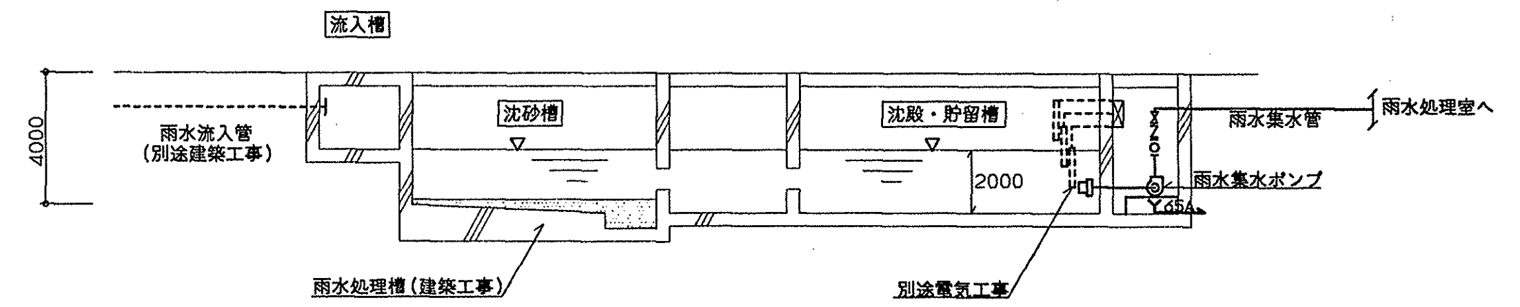
4 | 雨水处理設備系統図
