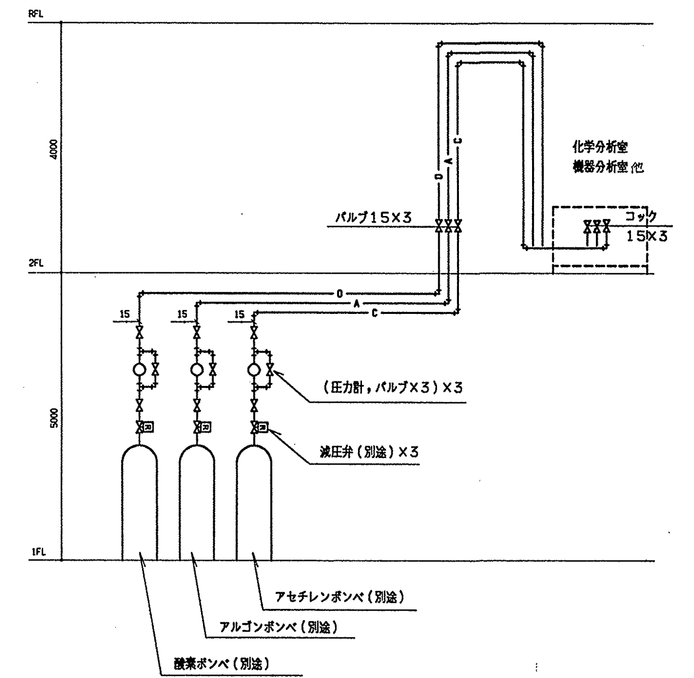
特殊ガス系統図
