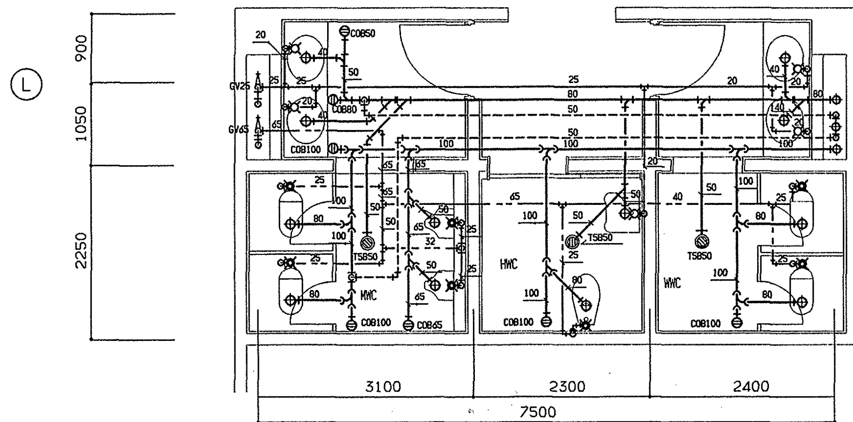
01 2階WC(2)平面詳細図
