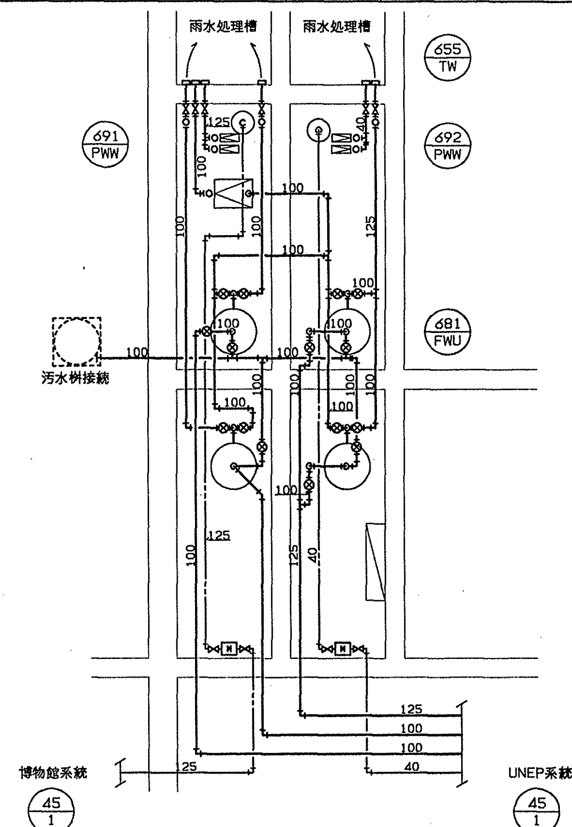
5 雨水処理室平面詳細図 1/100
