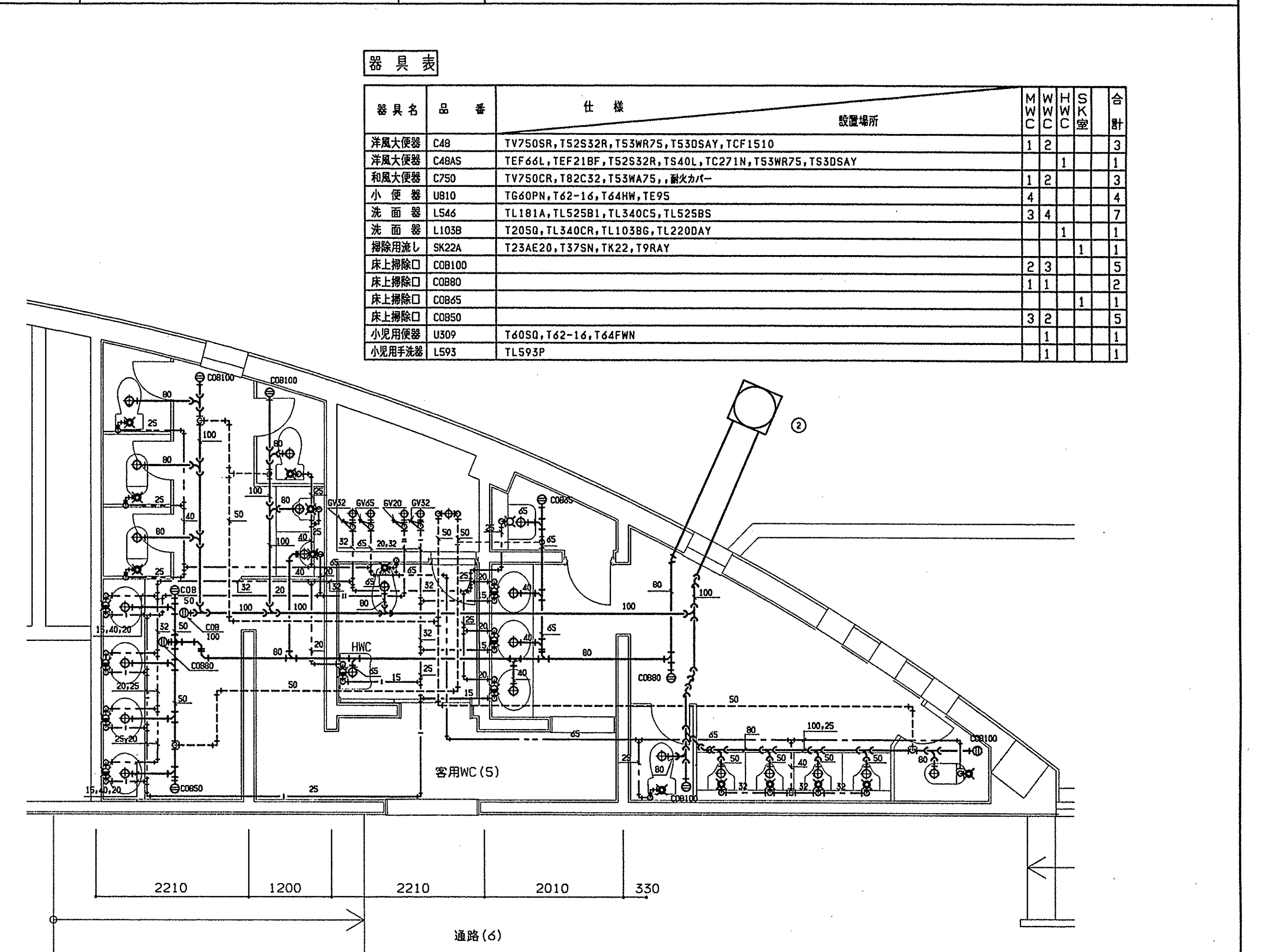
02 1階客用WC(5)平面詳細図 1/50
