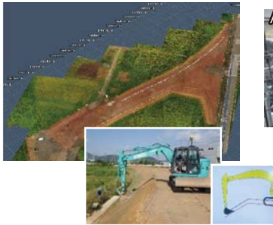
ICTバックホウによる法面整形 (仕上げ形状データを機械に入れて自動操作)
