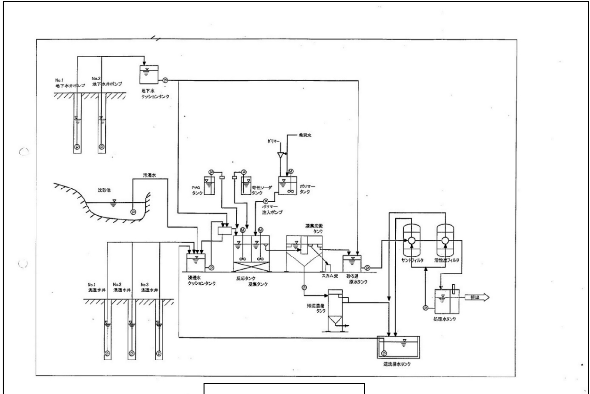
水処理施設の概念図
