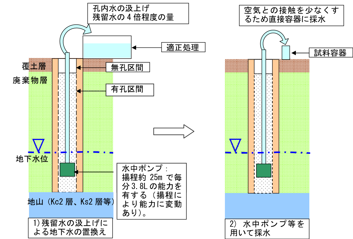
図-2.4.1 浸透水・地下水の採水手順
