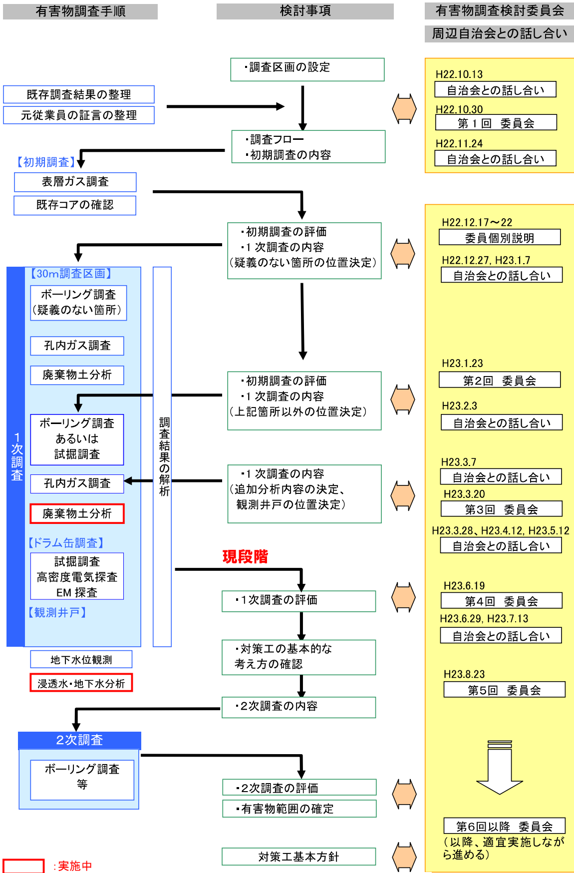
図-1.1 有害物調査の進め方
