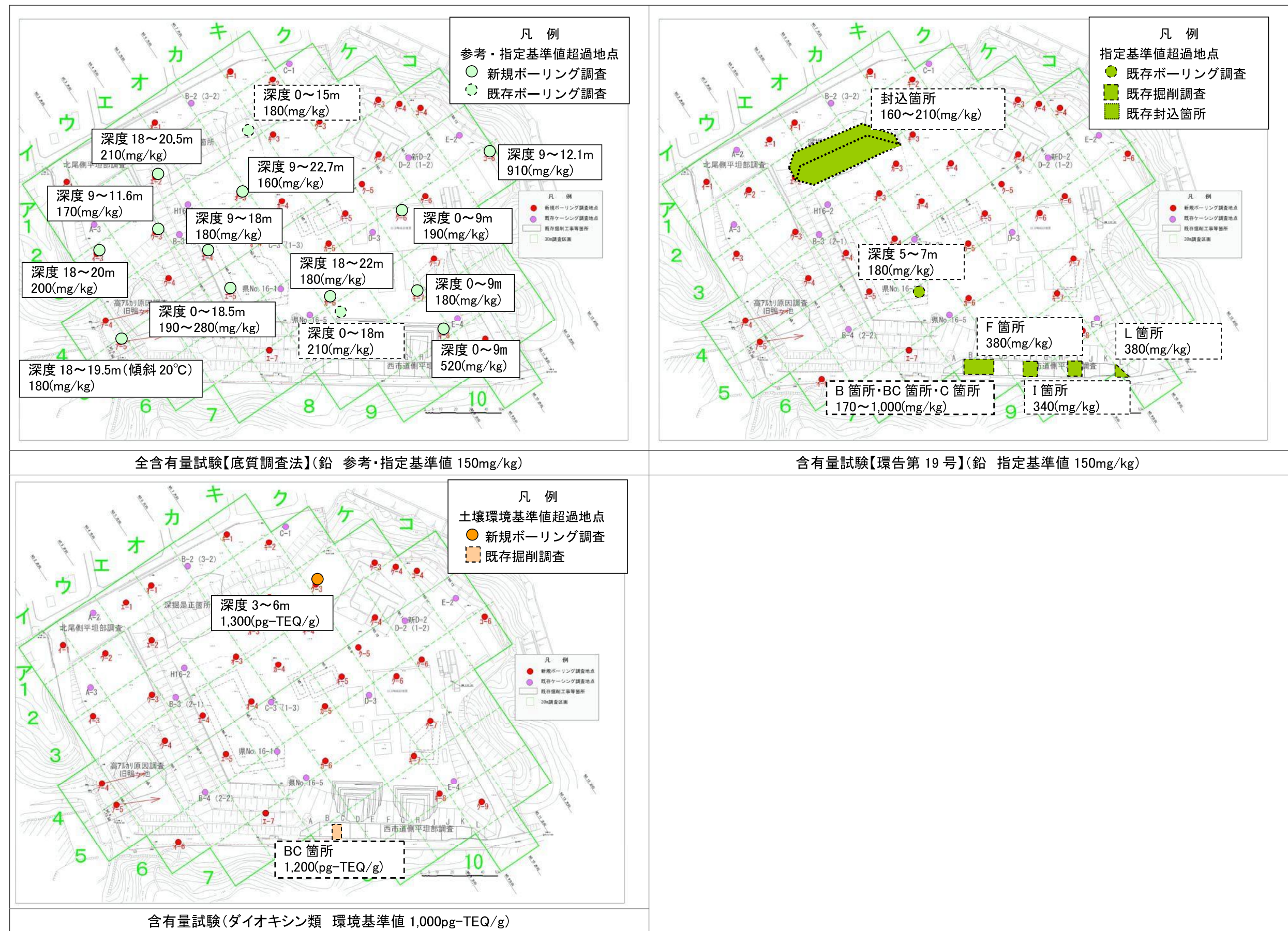
図-2.3.5 廃棄物土分析結果図（含有量試験）
