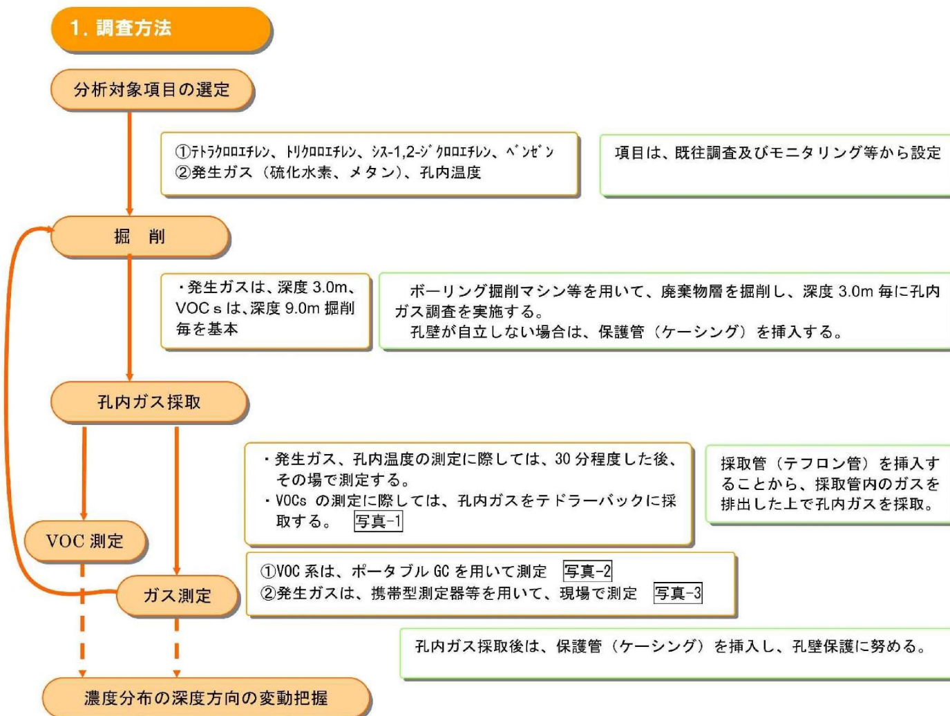
図-2.2.1 孔内ガス調査フロー
