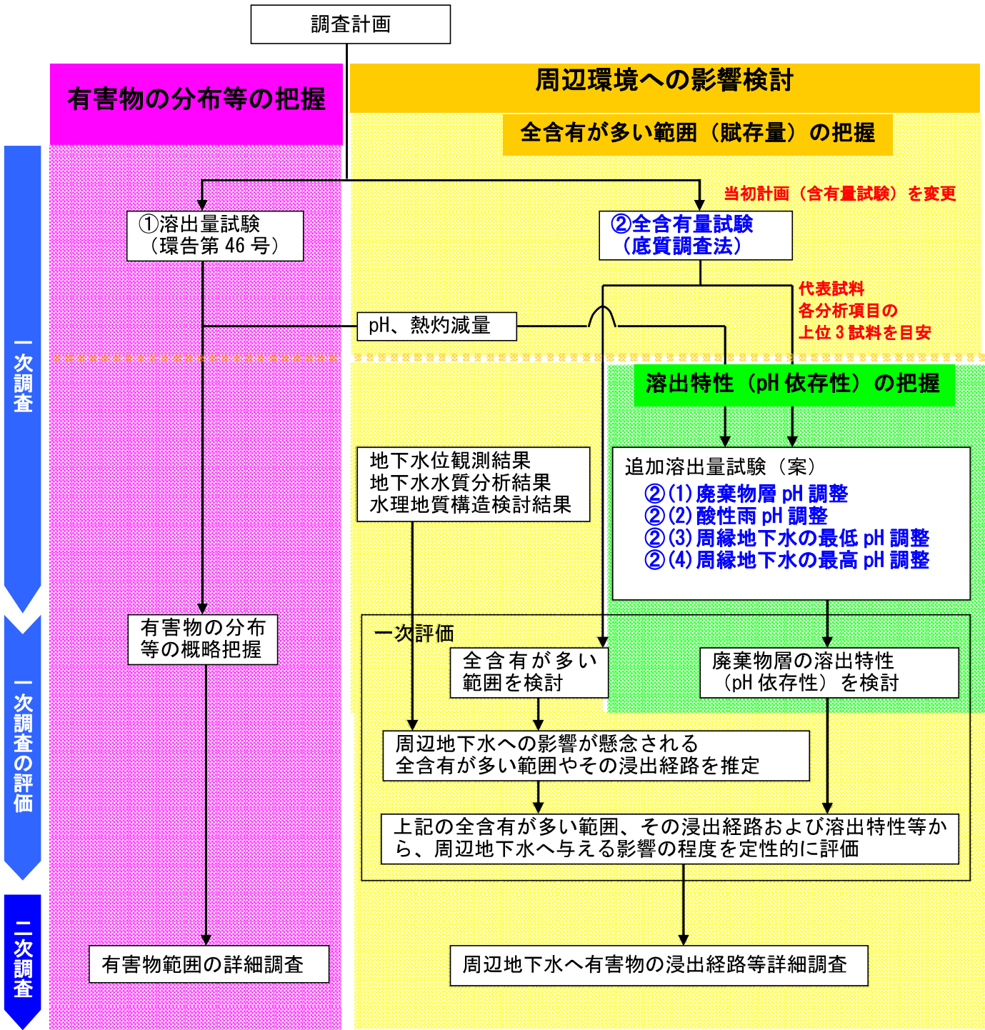
図-2.3.2 廃棄物土分析フロー図
