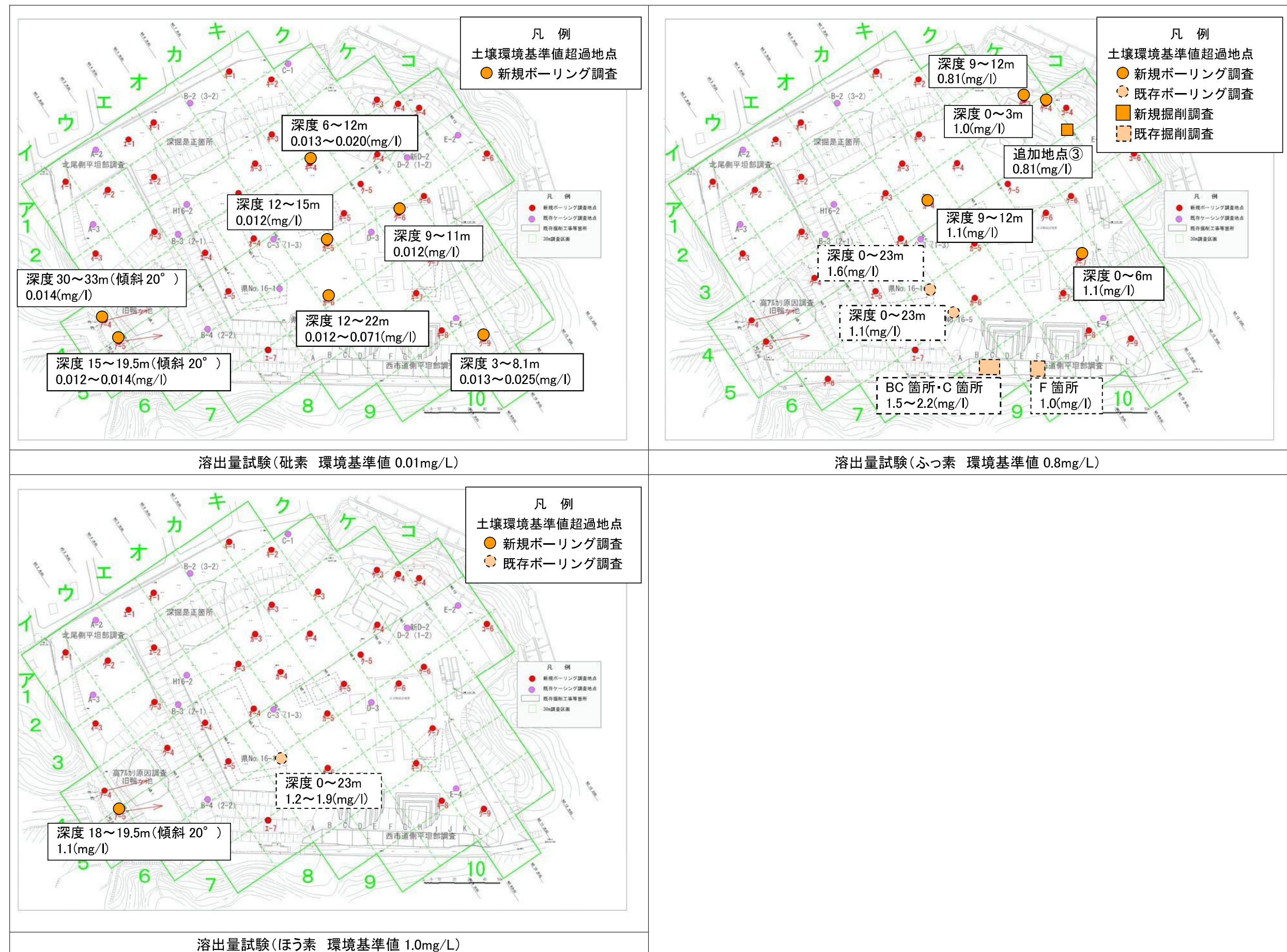
図-2.3.4 廃棄物土分析結果図（溶出量試験 重金属等）
