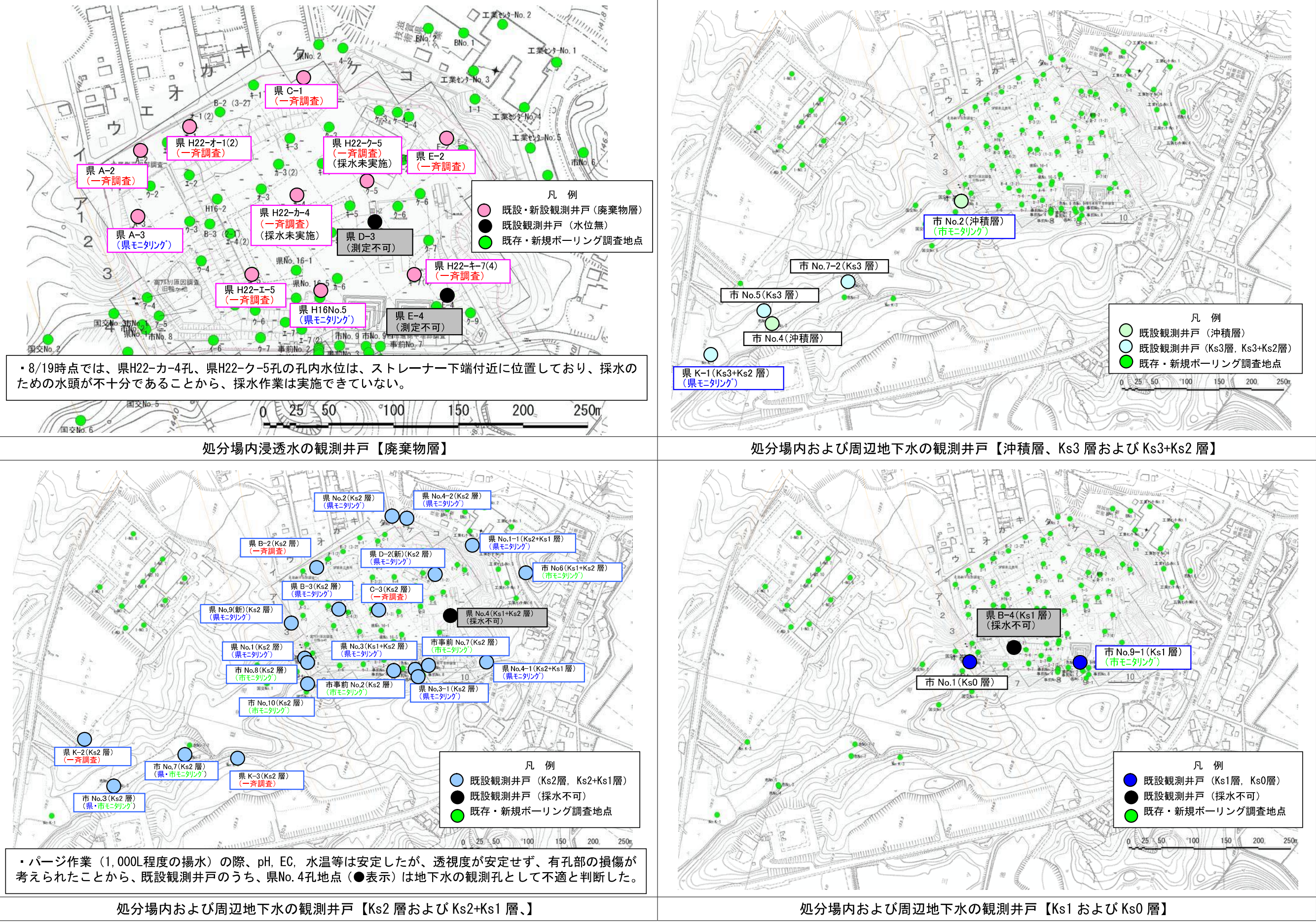
図-2. 4. 2 処分場内浸透水・場内および周辺地下水の調査地点位置図
