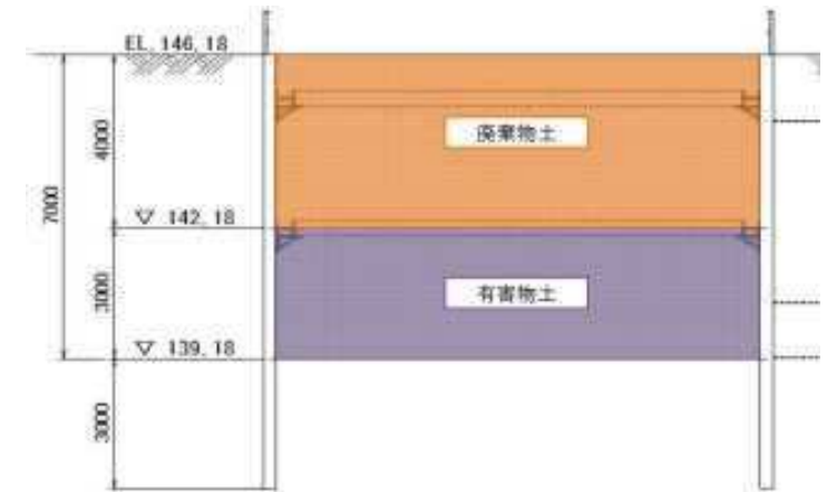
図3 A-3区画掘削断面図
