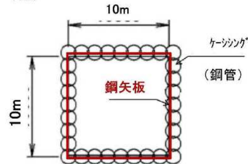
図5 オールケーシング工法配置 平面図
