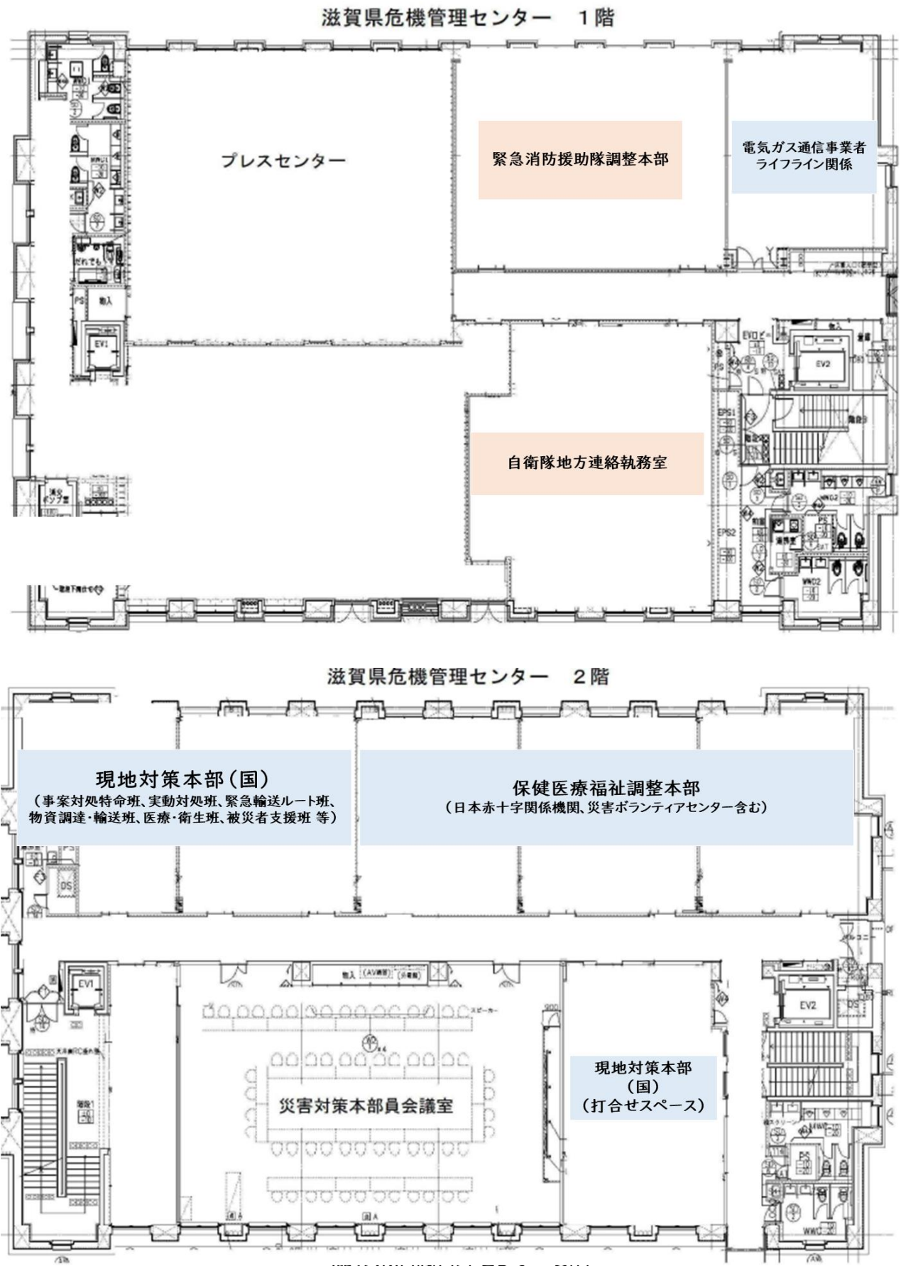
(図一 1) (災害時危機管理センター配置図 (案))
