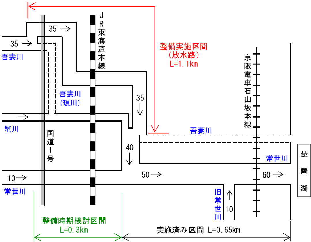
常世川・吾妻川 計画流量配分図
