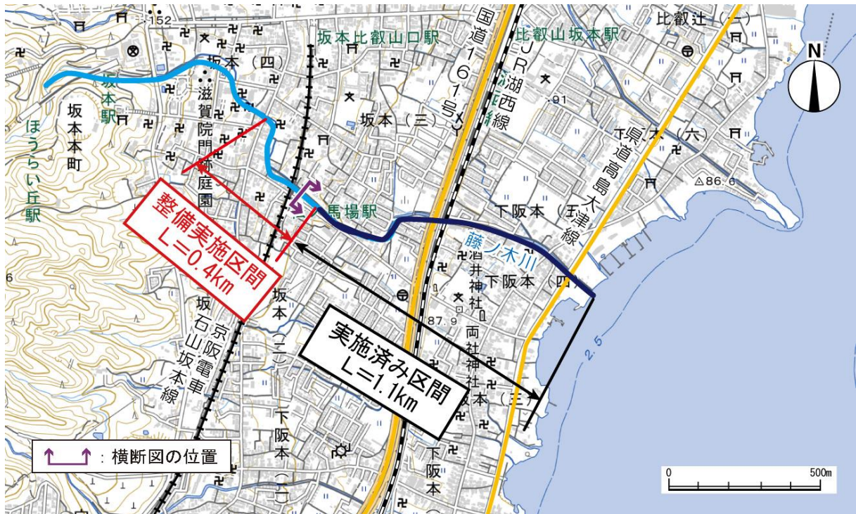
藤ノ木川平面図
