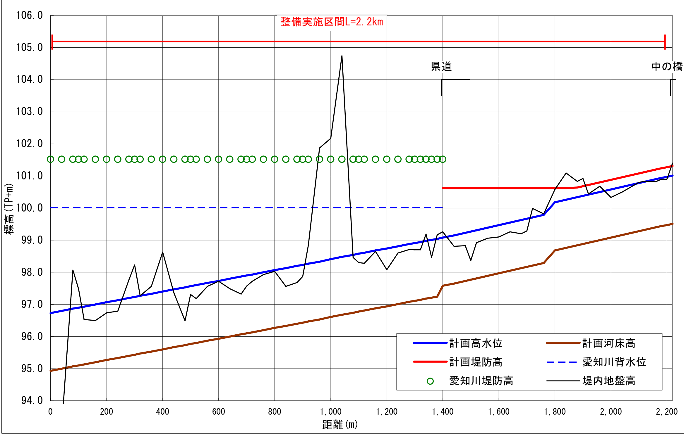
不飲川放水路縦断面図
