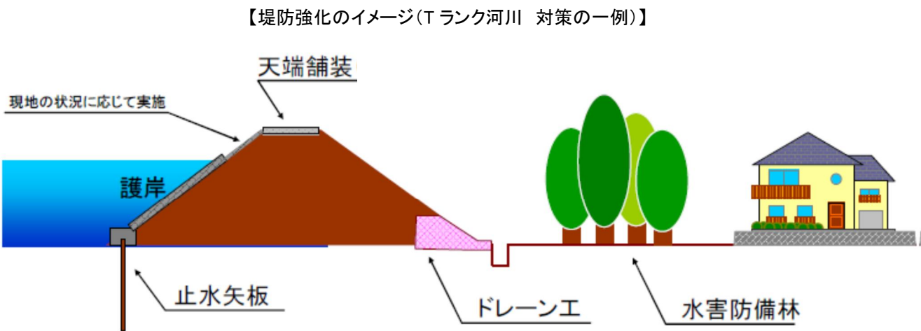
■堤防強化
