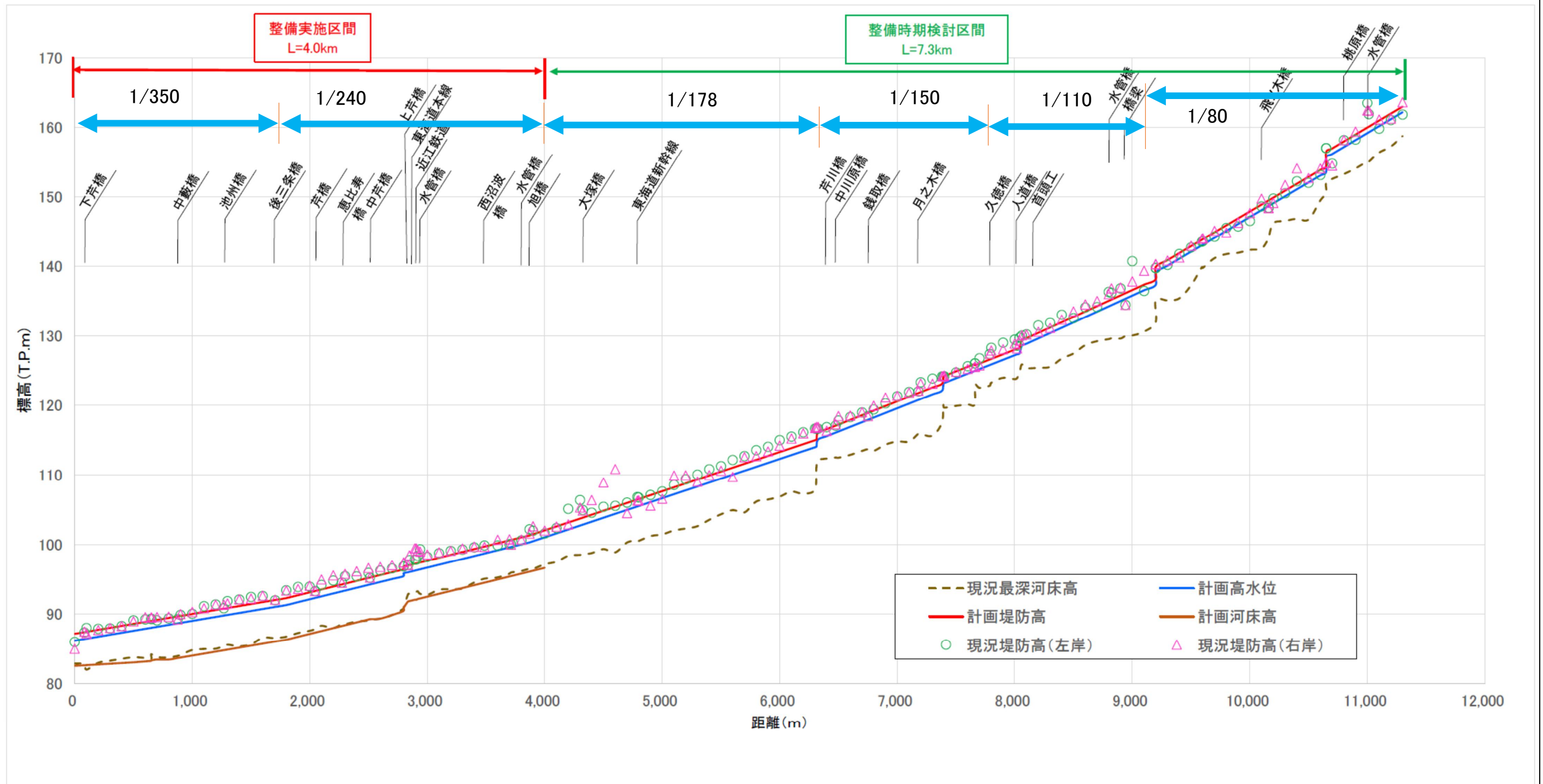
芦川計画縦断面
