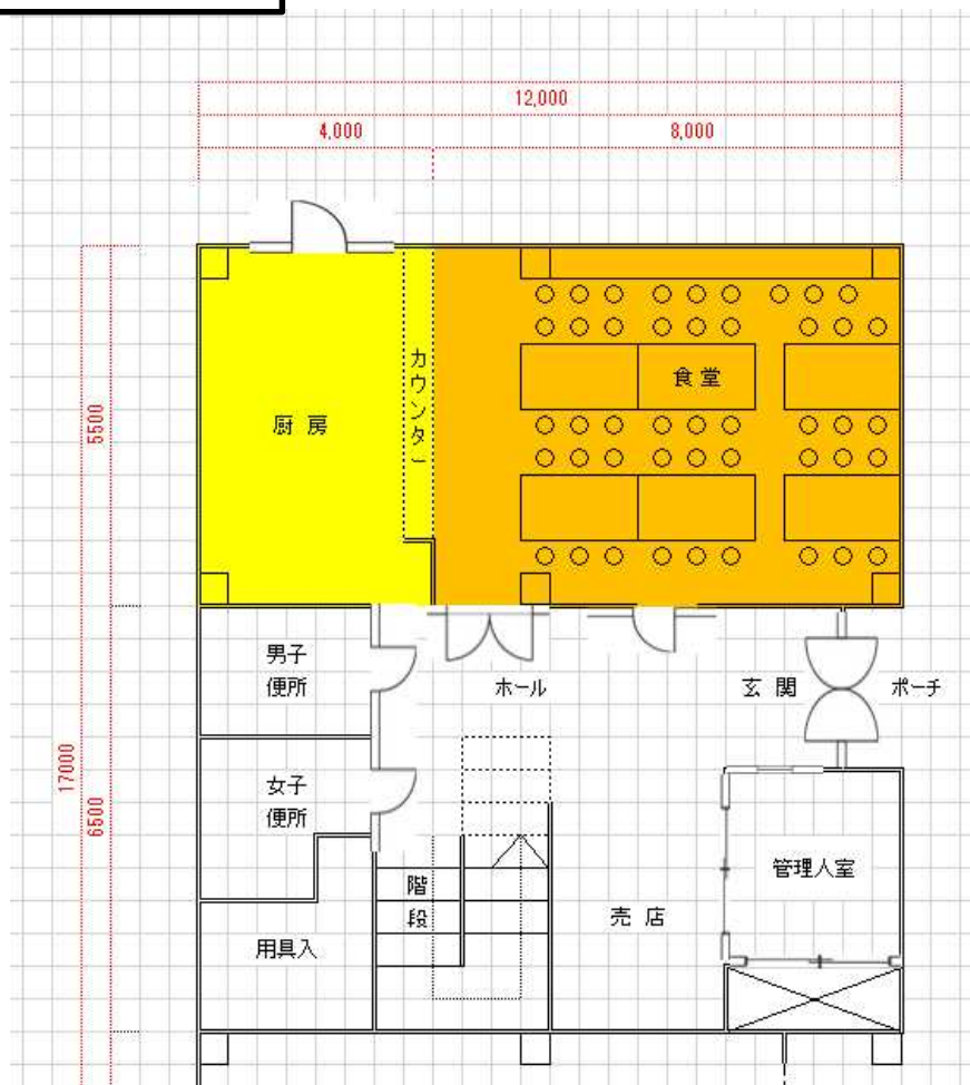
施設平面図
