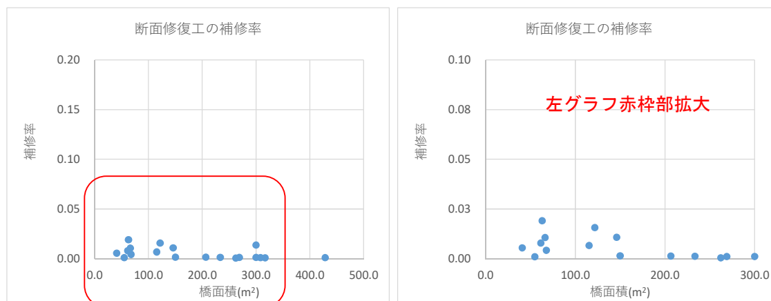
図 6-3 橋面積と断面修復修繕率の関係
