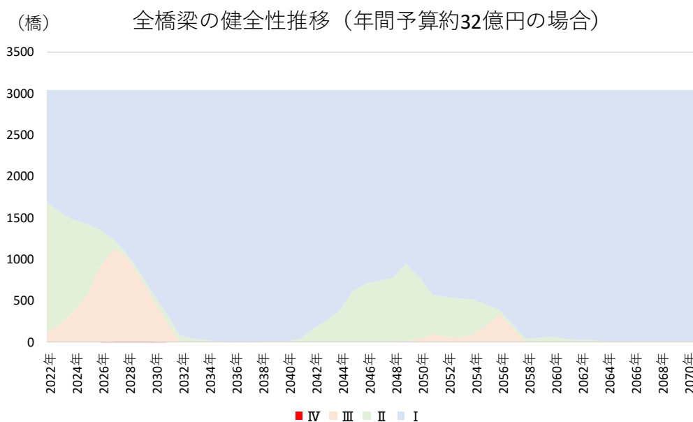
図 7-9 健全性の推移
