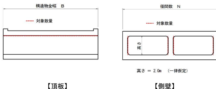
図 6-5 ボックスカルバートの表面積算出方法
