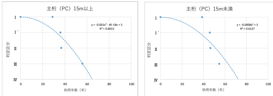
図 3-6 PC 橋主桁の劣化曲線
