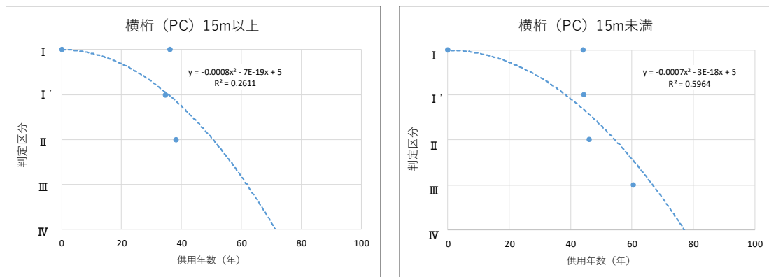
図 3-7 PC 橋横桁の劣化曲線
