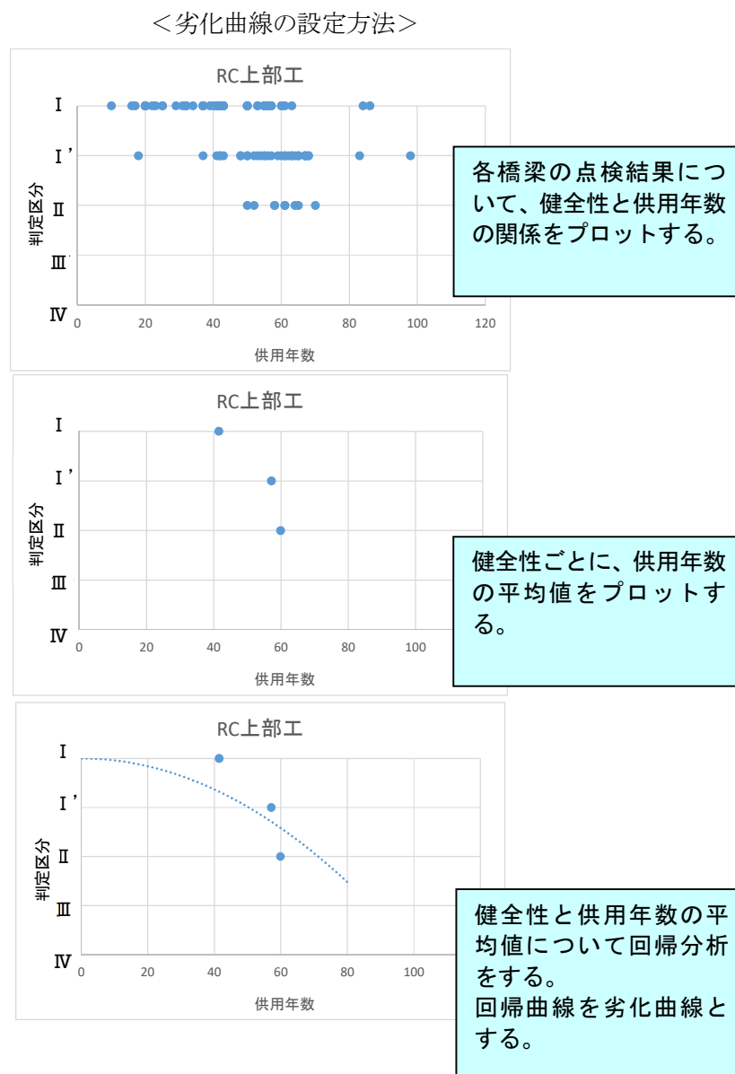
図 3-3 劣化曲線の設定方法
