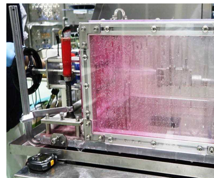
ノズルによる洗浄試験の様子
