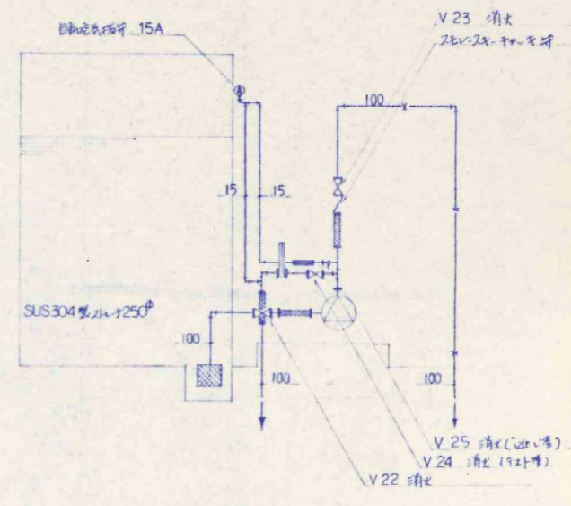
排水ポンプ系統図
