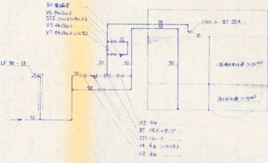
受水槽ポンプ室の配管図 (詳細図)
