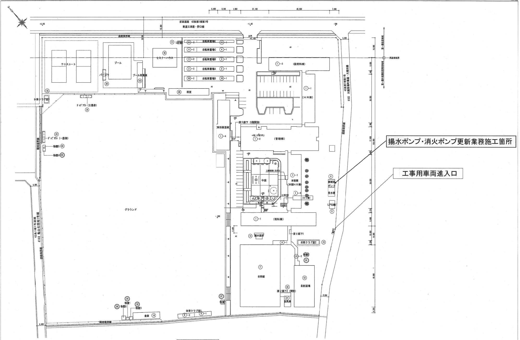
配置図 1/500
