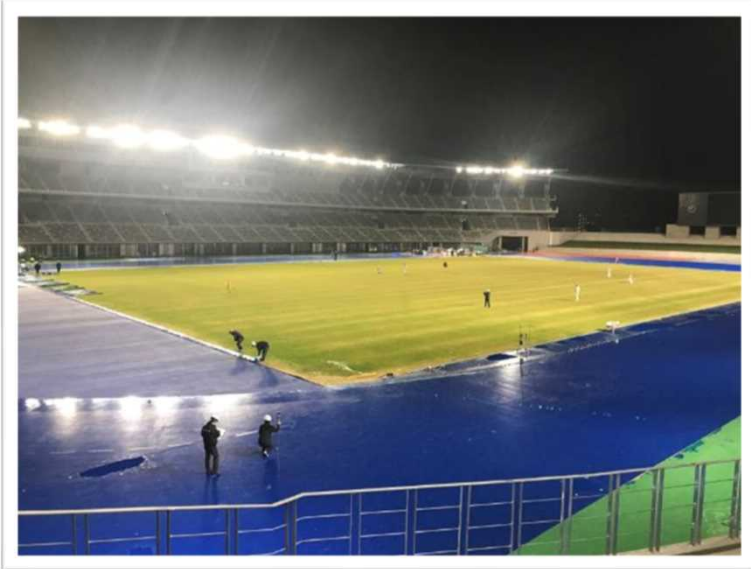
金亀公園第Ⅰ種陸上競技場のLED照明 と キュービクル盤
