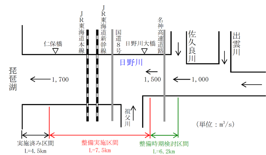
日野川の計画流量配分図
