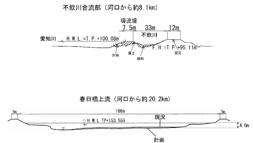
横断面図
