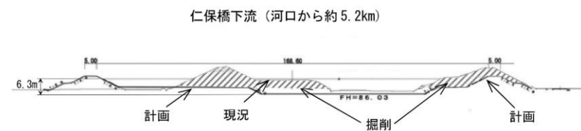
横断図
