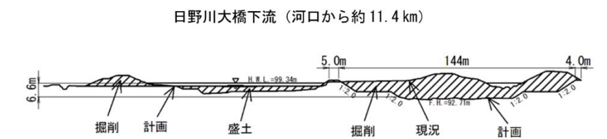
横断図
