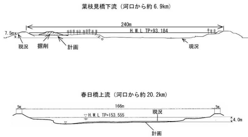
横断面図
