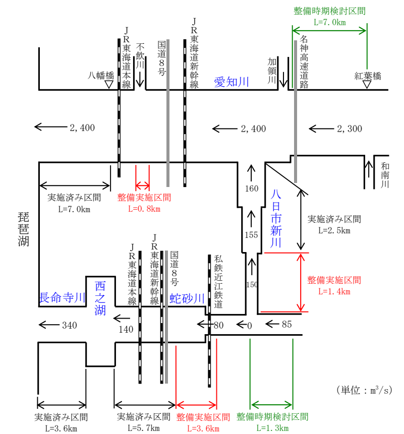
愛知川・長命寺川・蛇砂川・八日市新川の計画流量配分図
