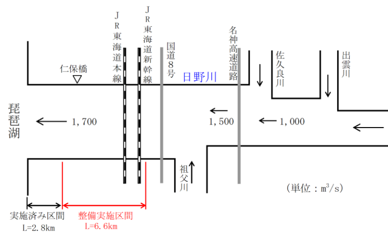
日野川の計画流量配分図
