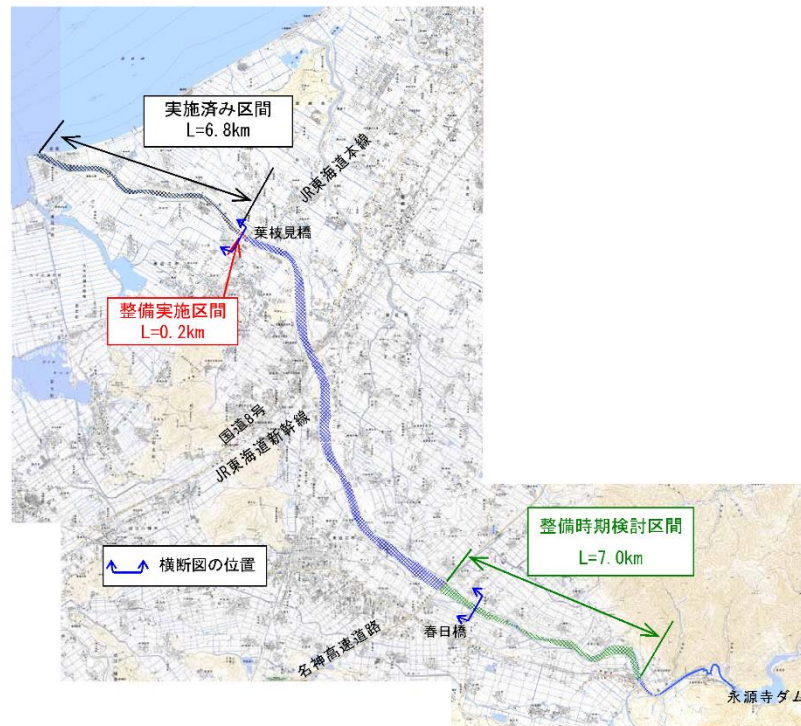
愛知川平面図
