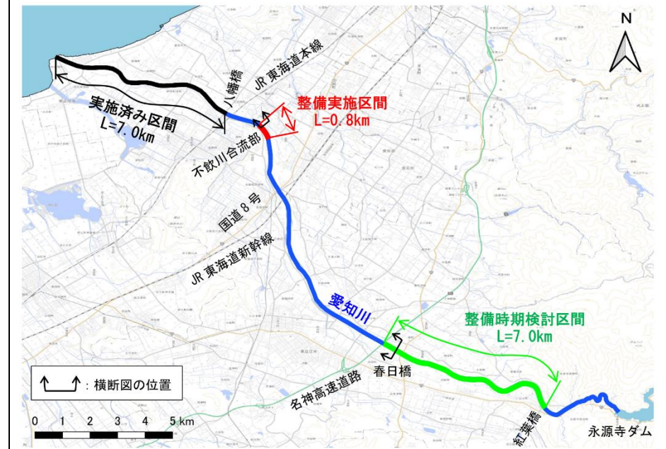
愛知川平面図
