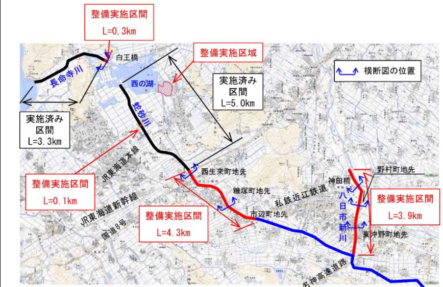
長命寺川(蛇砂川)・八日市新川平面図
