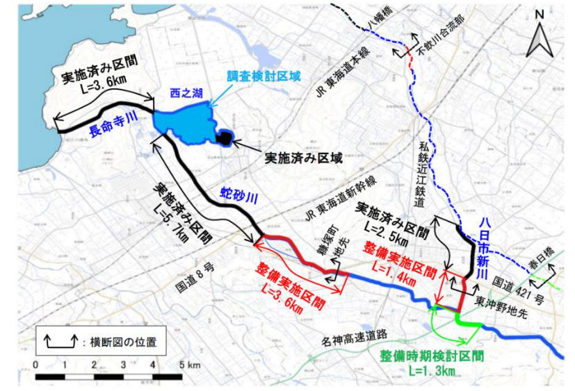
長命寺川・蛇砂川・八日市新川平面図
