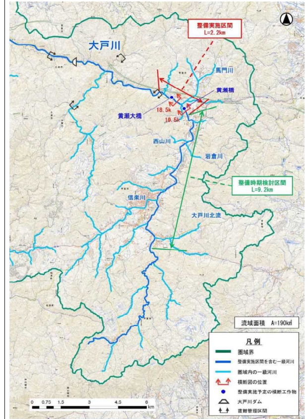
大戸川上流区間平面図
