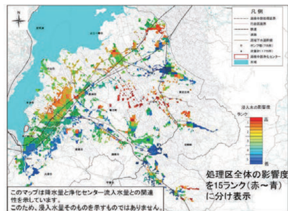
図2 取組対策例:不明水影響度マップ
