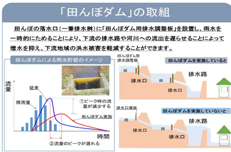
【図表-53】「田んぼダム」の取組について
