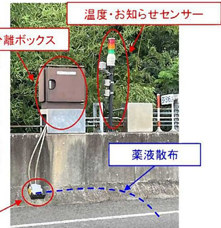
薬剤散布式消雪設備 整備イメージ
