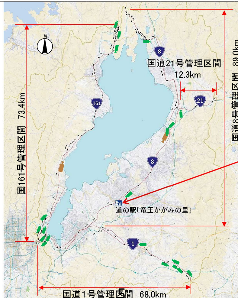
車両停滞を感知しアラーム発報
