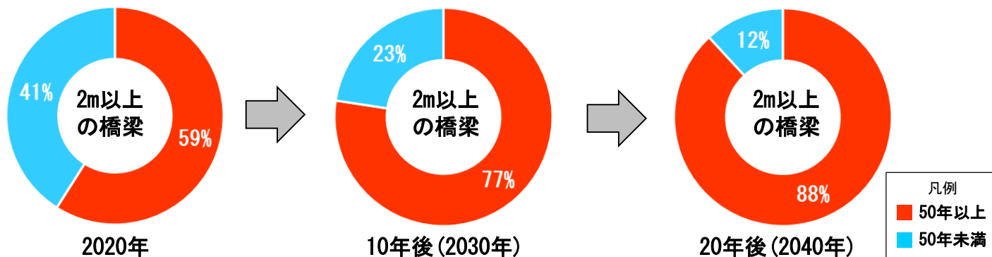
■滋賀県における建設後50年以上経過した橋梁の割合の変化
