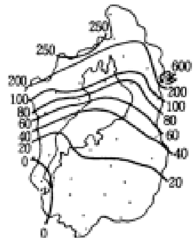
昭和27年2月6日9時 積雪分布図 単位：cm
