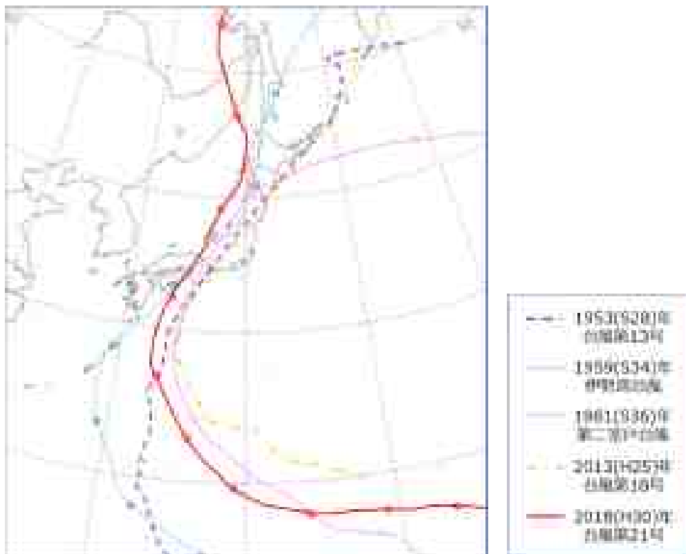
顕著な台風の経路図
