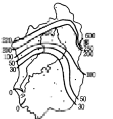
昭和27年2月18日9時 積雪分布図 単位：cm
