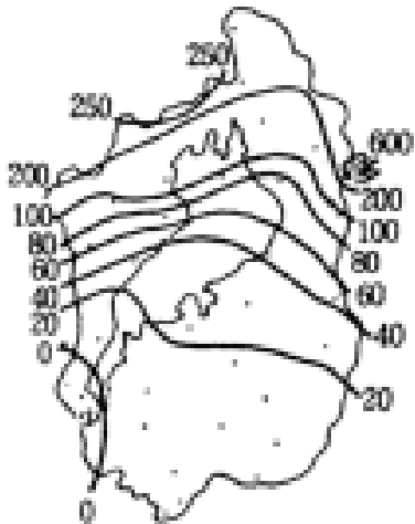
昭和52年 2 月 6 日 9 時 積雪分布図 単位：cm
