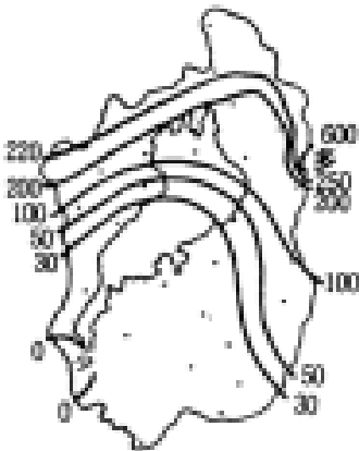
昭和52年 2 月18日 9 時 積雪分布図 単位：cm
