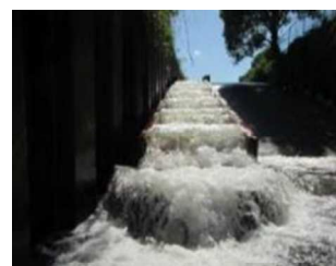
落差工に設置した魚道
