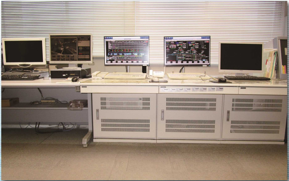
水口浄水場中央監視システム
