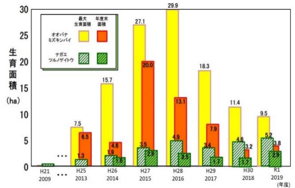
侵略的外来水生植物 2 種の生育面積の経年変化 (平成 21 年度～令和元年度)
