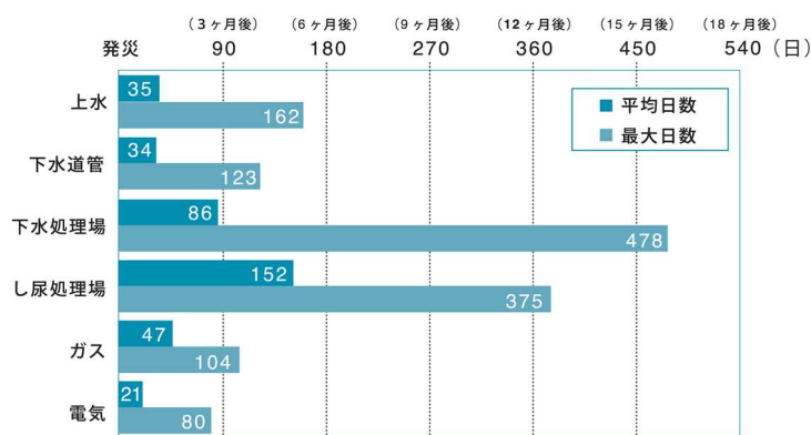
図 1-2 東日本大震災被災自治体におけるライフライン別の仮復旧までの日数 (回答：29 自治体) 出典：日本トイレ研究所
