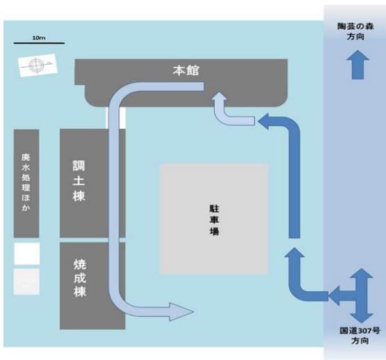
敷地内建物レイアウトと動線（例）
