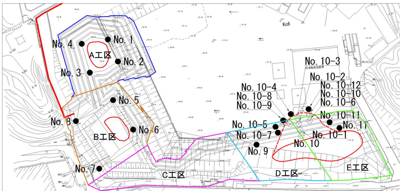
図-1 事前調査ボーリング全体図
