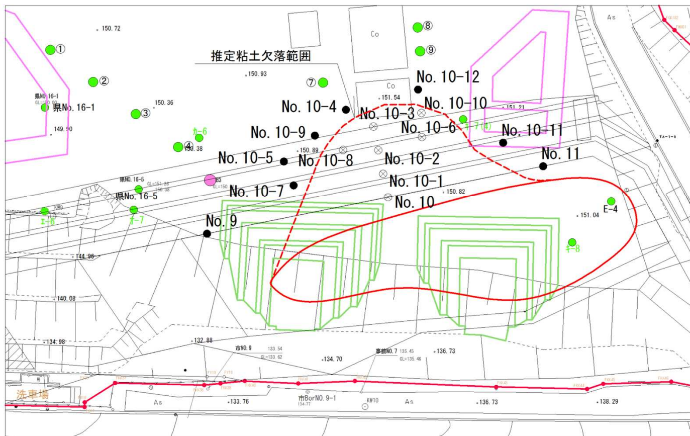
図-2 D・E工区詳細図
