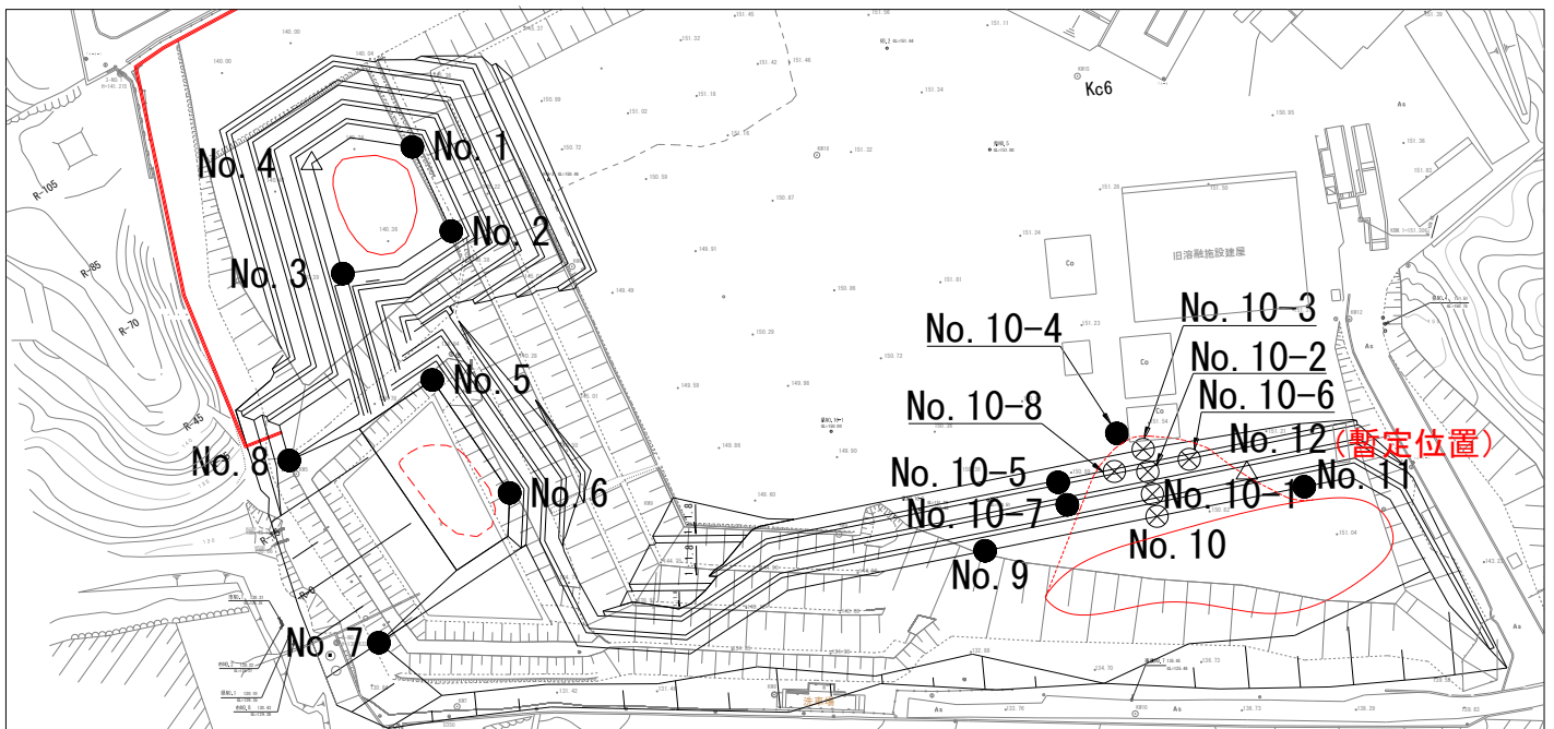
図-1 事前調査ボーリング全体図
