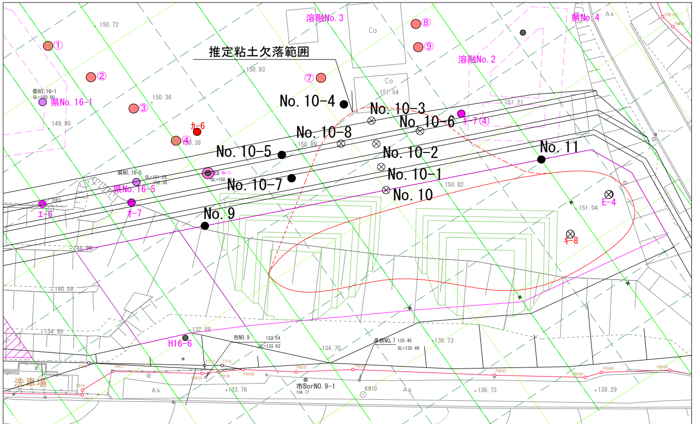
図-2 D・E工区詳細図
