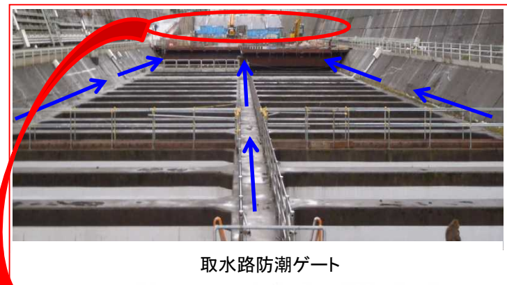
取水路防潮ゲート (出典:高浜原子力規制事務所保安検査官撮影の写真の一部加筆)
