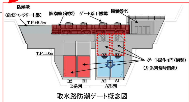
取水路防潮ゲート (出典:高浜原子力規制事務所保安検査官撮影の写真の一部加筆)
