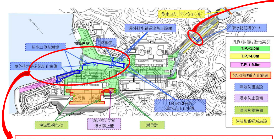
取水路防潮ゲート (出典:高浜原子力規制事務所保安検査官撮影の写真の一部加筆)
