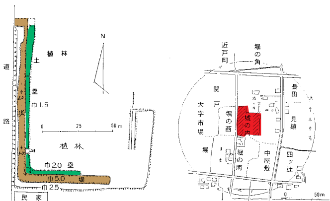
大原氏館跡平面図
