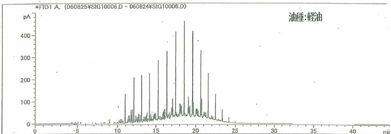
TPH試験(GC/FID)ーガスクロチャート図
