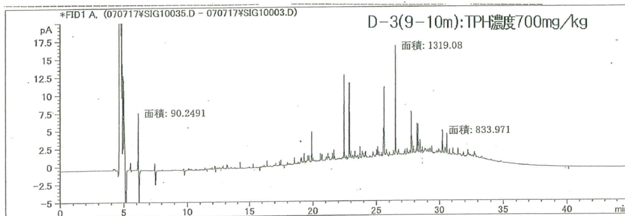
TPH試験(GC/FID)-ガスクロチャート図
