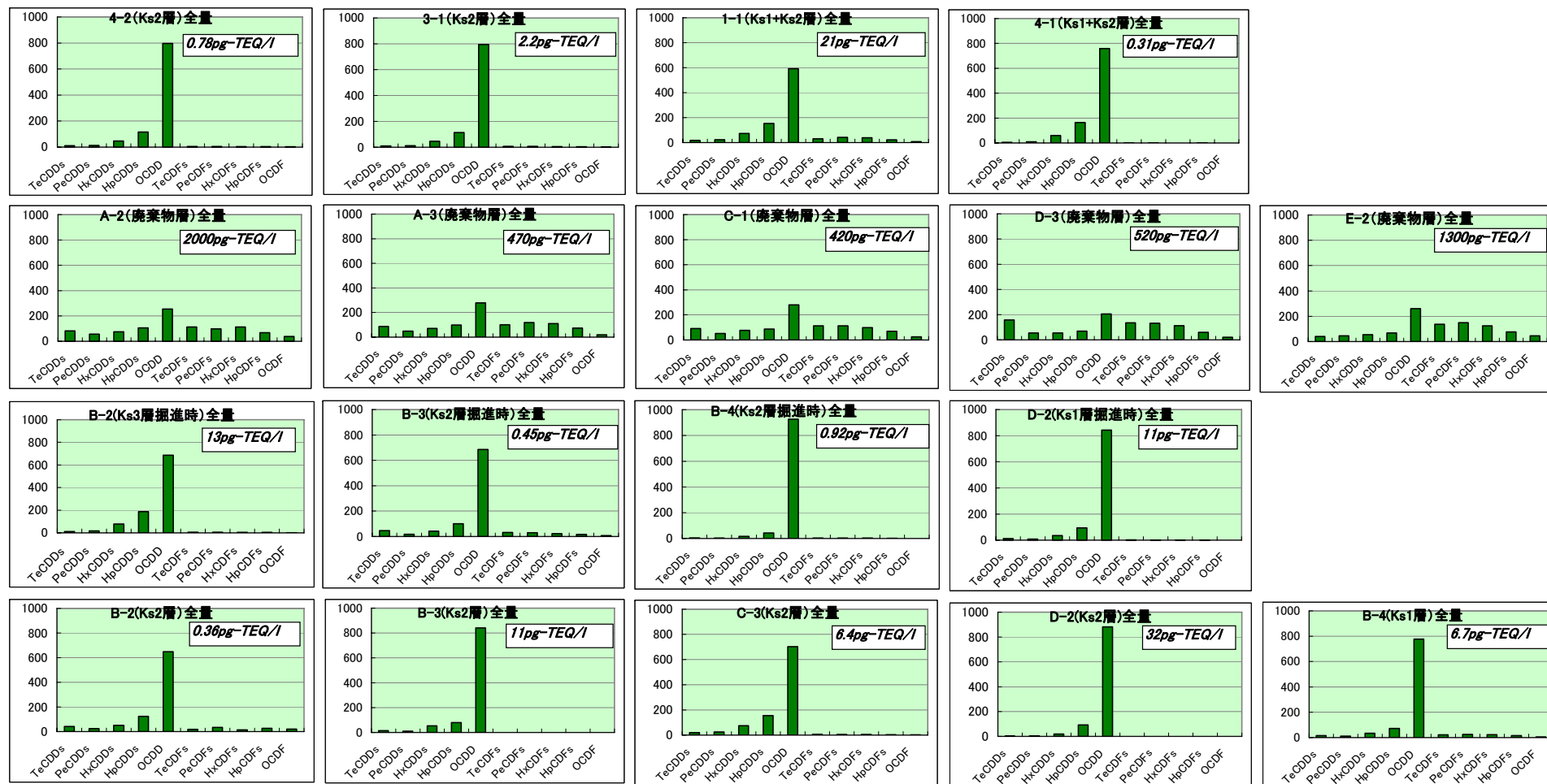
地下水・浸透水のダイオキシン類のパターン図(パターンは同族体実測濃度換算(%))。濃度は毒性換算濃度。)
