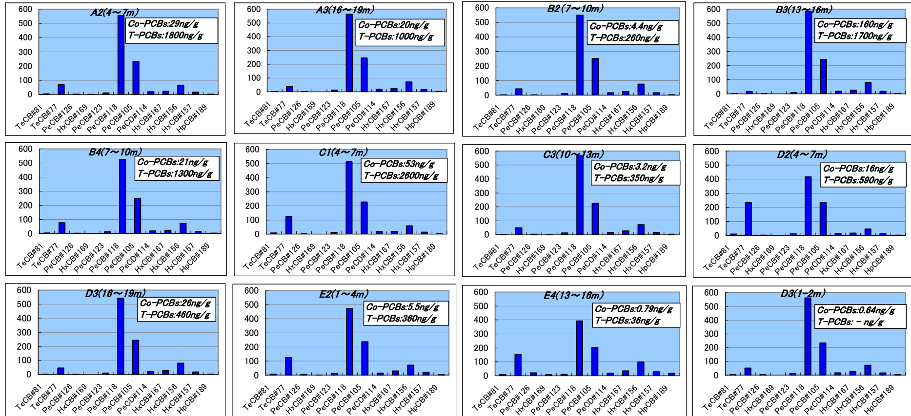
処分場内廃棄物土のプロナ-PCBsのパターン図(パターンは異性体実測濃度換算(%))。濃度はプロナ-PCBsと総PCBs実測濃度。
