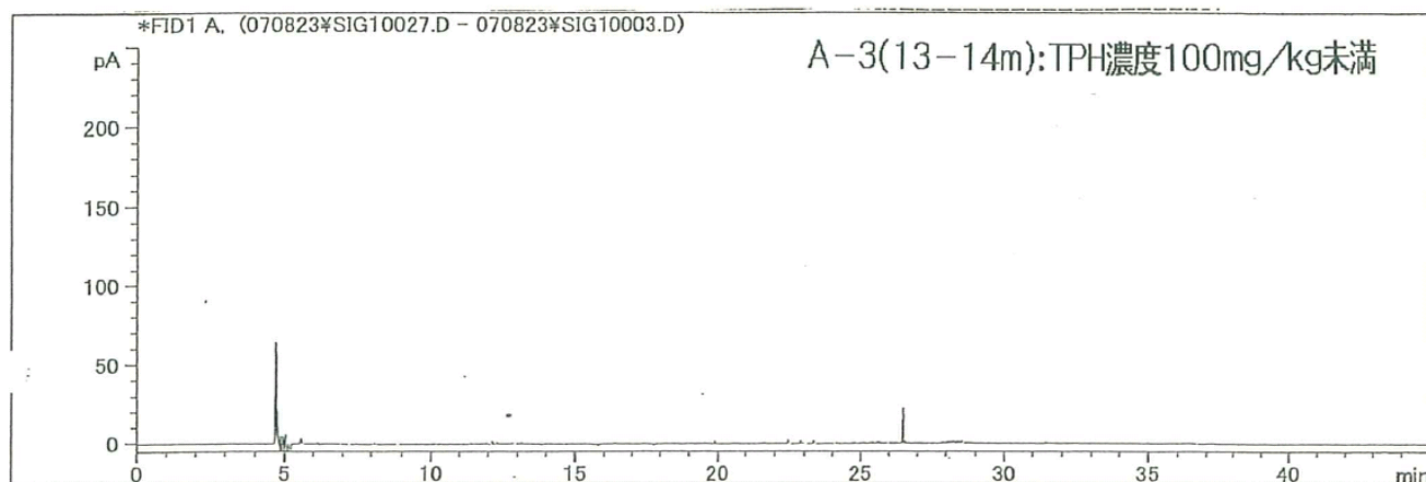
TPH試験(GC/FID)-ガスクロチャート図
