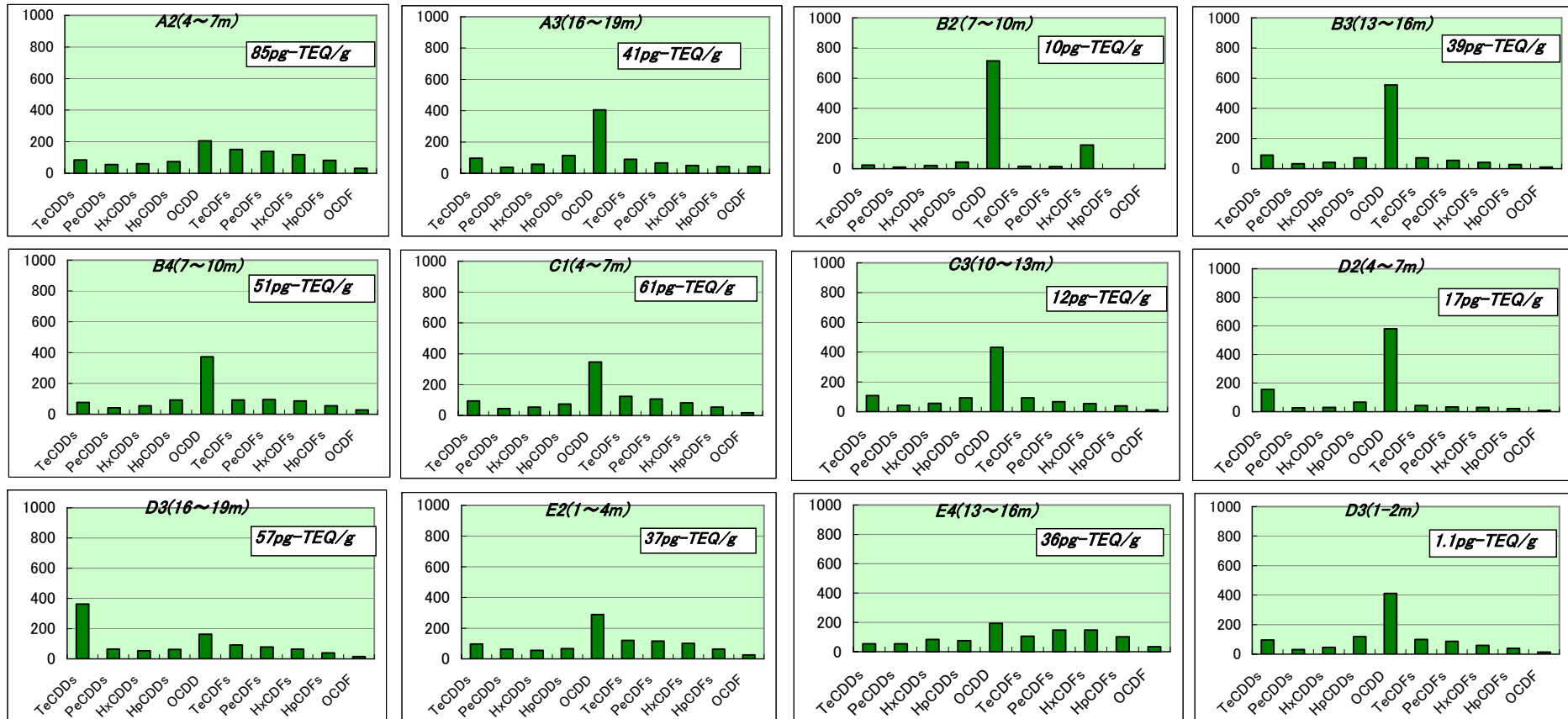
処分場内廃棄物土のダイオキシン類のパターン図(パターンは同族体実測濃度換算(%))。濃度は毒性換算濃度。)
