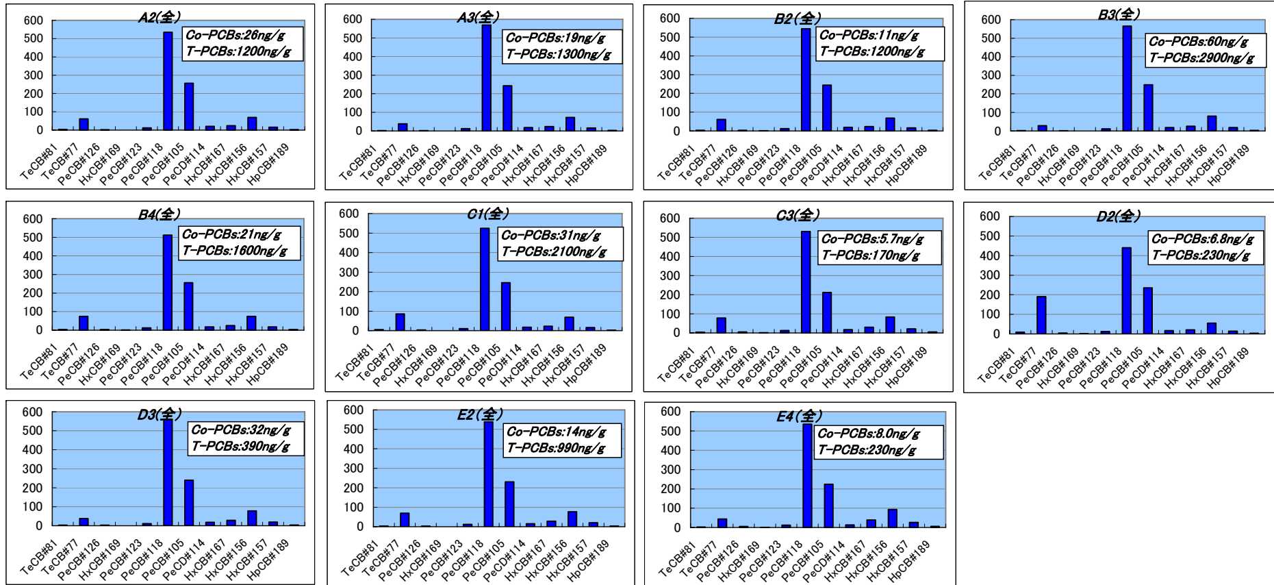
処分場内廃棄物土のプロナ-PCBsのハターン図(ハターンは異性体実測濃度換算(%))。濃度はプロナ-PCBsと総PCBs実測濃度。)
