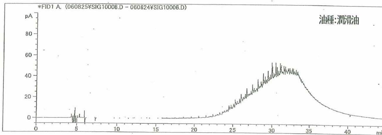
TPH試験(GC/FID)-ガスクロチャート図
