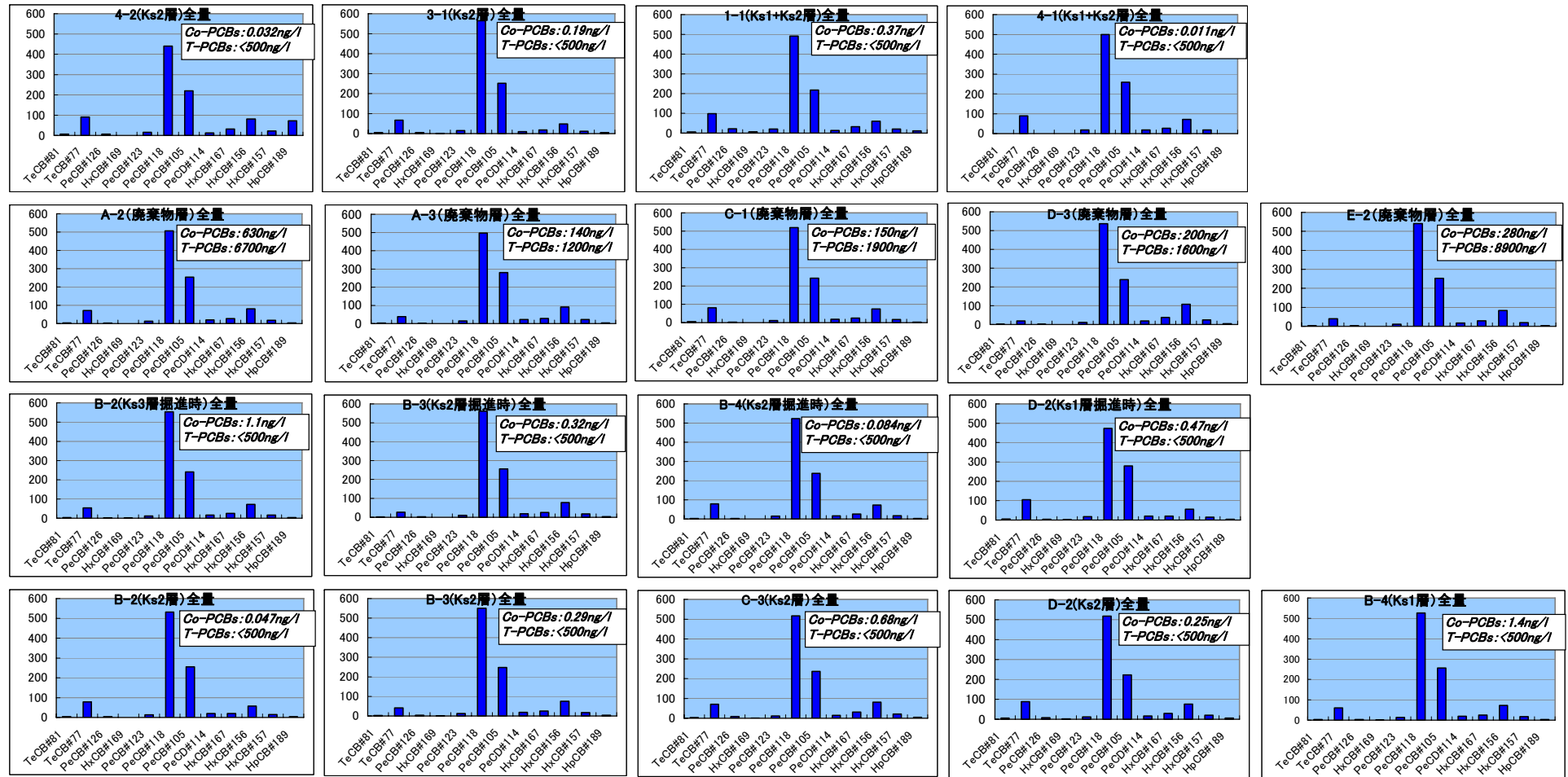
地下水・浸透水のコプラナーPCBsのパターン図(パターンは異性体実測濃度換算(%))。総PCBs(T-PCBs)もあわせて表記。
