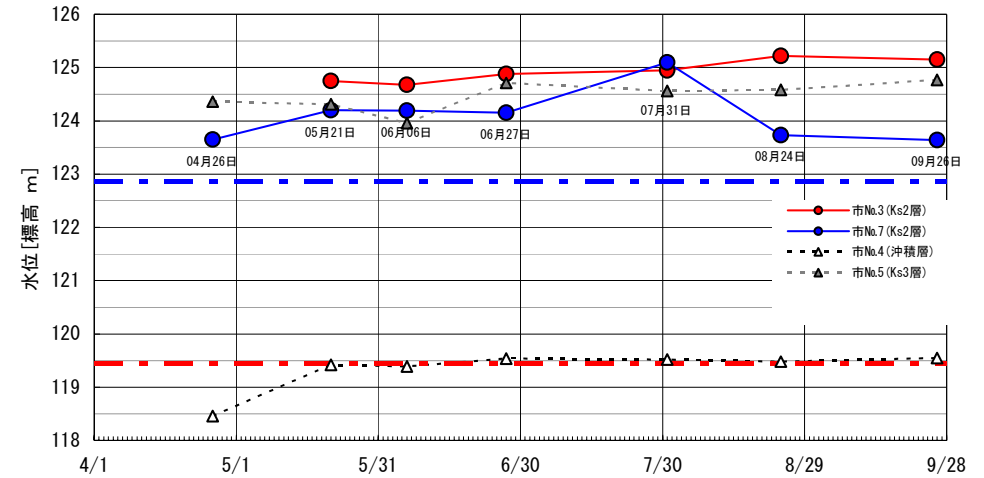
図2.1.5 市No.3と市No.7のKs2帯水層 地下水位の変化
