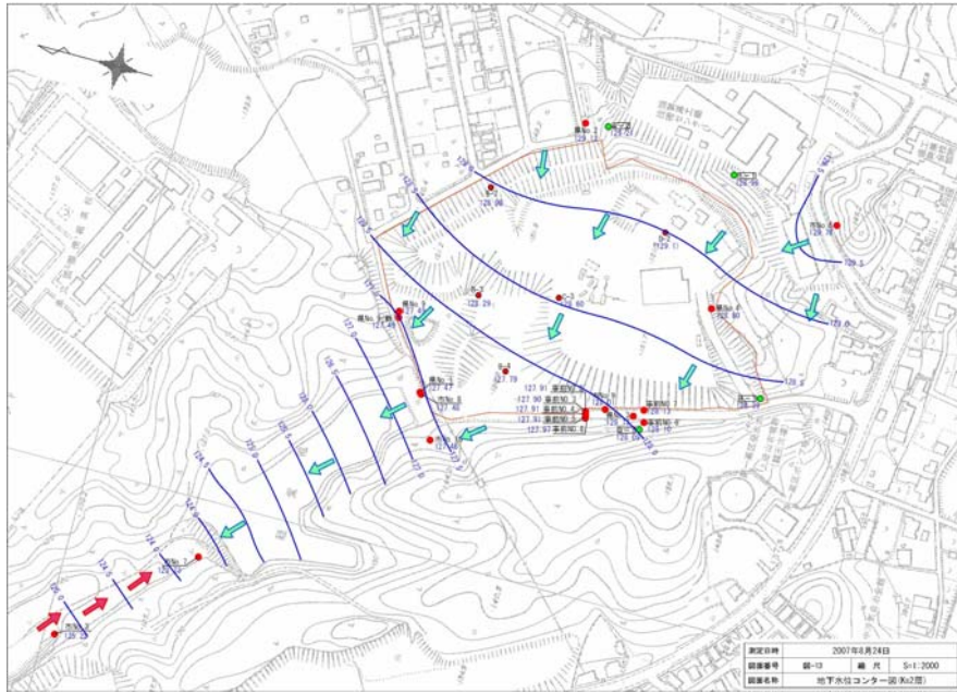
図2.1.4 (2) Ks2帯水層の地下水位等高線図 (平成19年8月24日測定) ←: 地下水位等高線に直交する流動方向 (推定)
