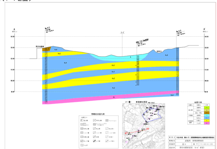
図 1 (2) 想定地質断面図〔A A'断面〕
