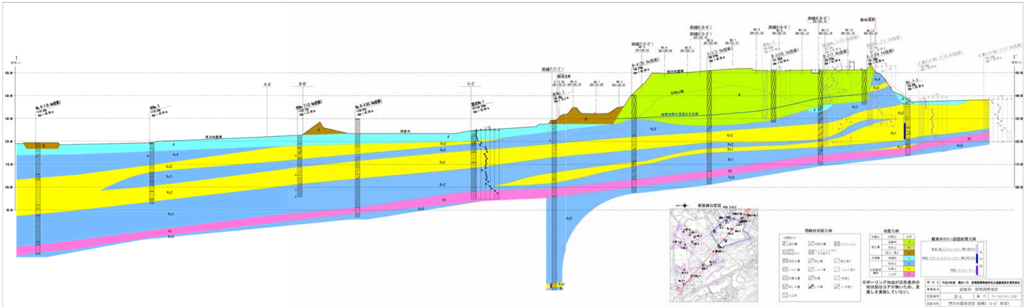
図 1 (1) 想定地質断面図〔1 1'断面〕
