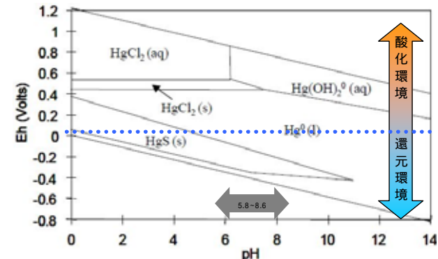
図2.1.2 Eh-pHダイアグラム(2)
