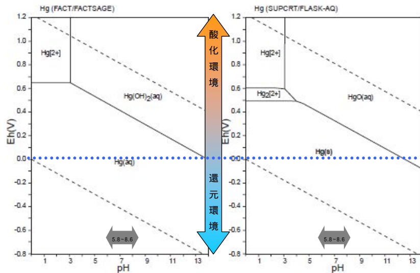
図2.1.1 Eh-pHダイアグラム(1)
