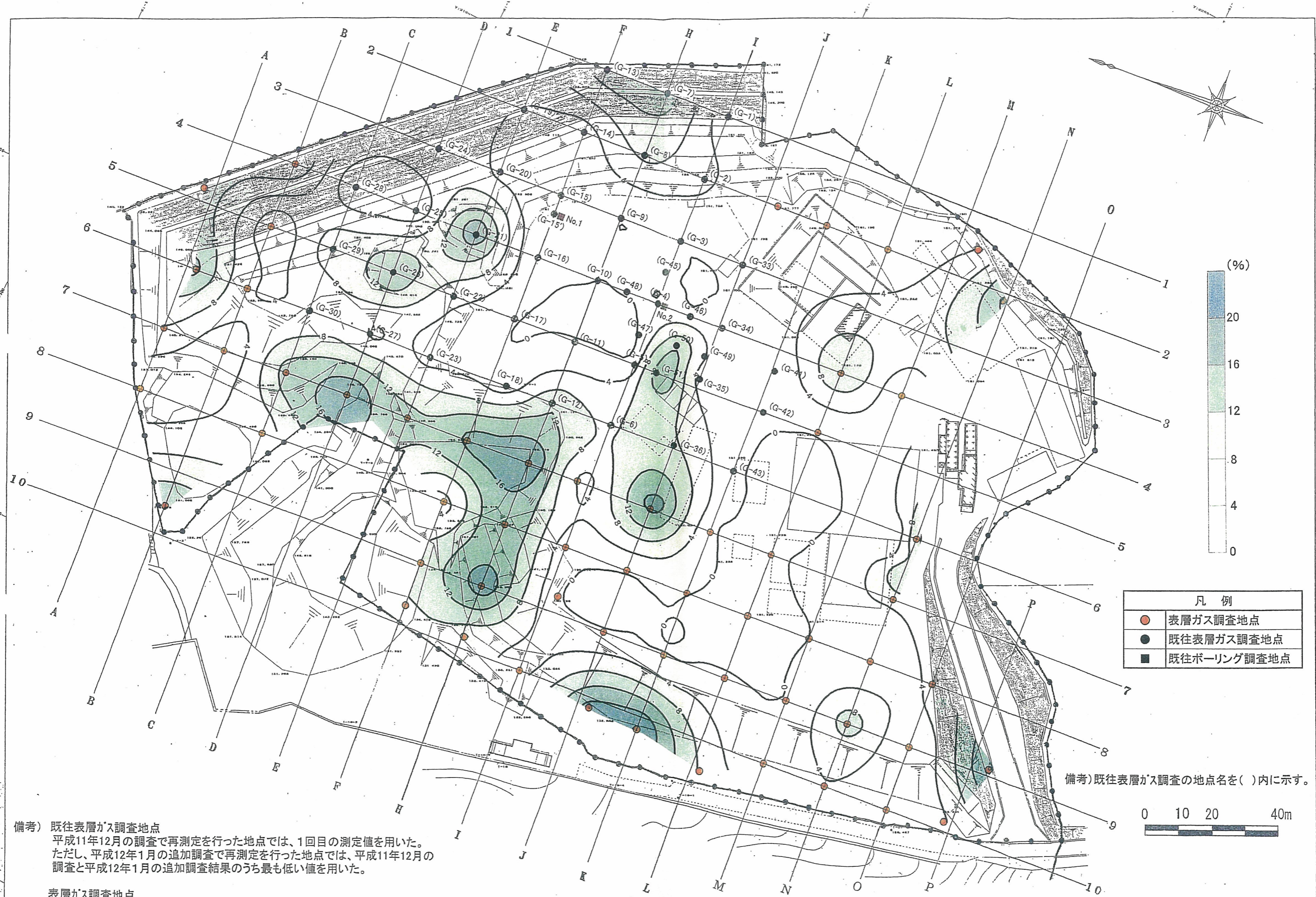
図 3 - 1 (2) 表層ガス濃度等高線図 (酸素)
