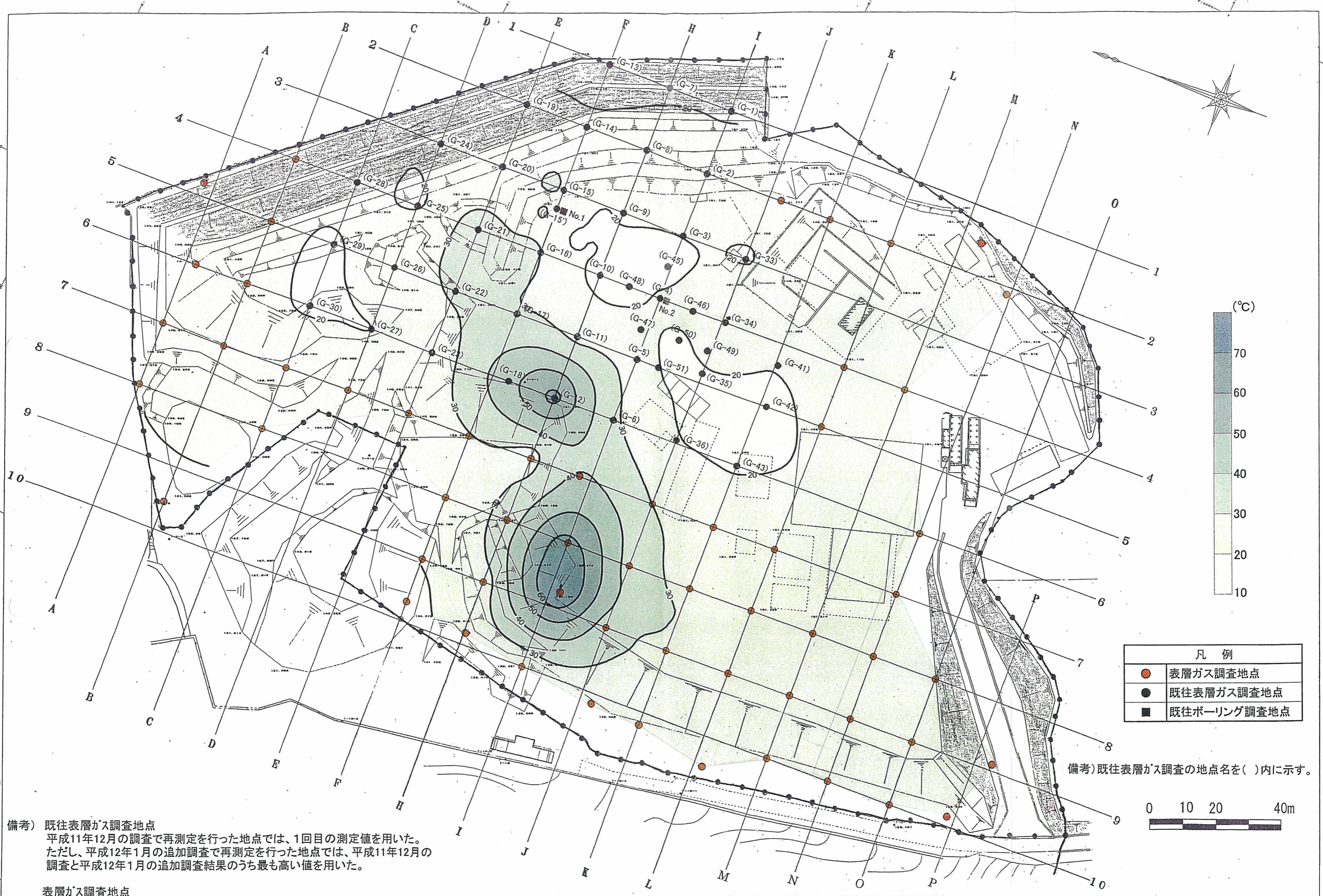
図2.6-1 孔内温度等高線図
