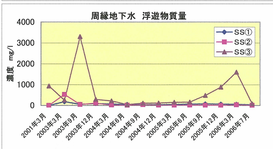
図2.3-5 周縁地下水経年変化3(県観測井戸No.1、No.2、No.3)
