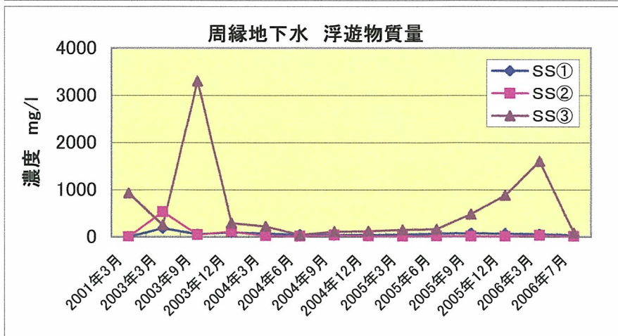
図2.3-3 周縁地下水経年変化1(県観測井戸No.1、No.2、No.3)
