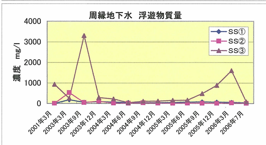
図2.3-4 周縁地下水経年変化2(県観測井戸No.1、No.2、No.3)
