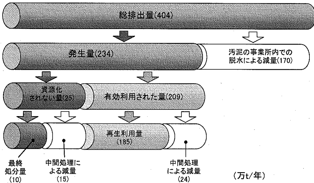
産業廃棄物の処理の概念図（平成19年度）
