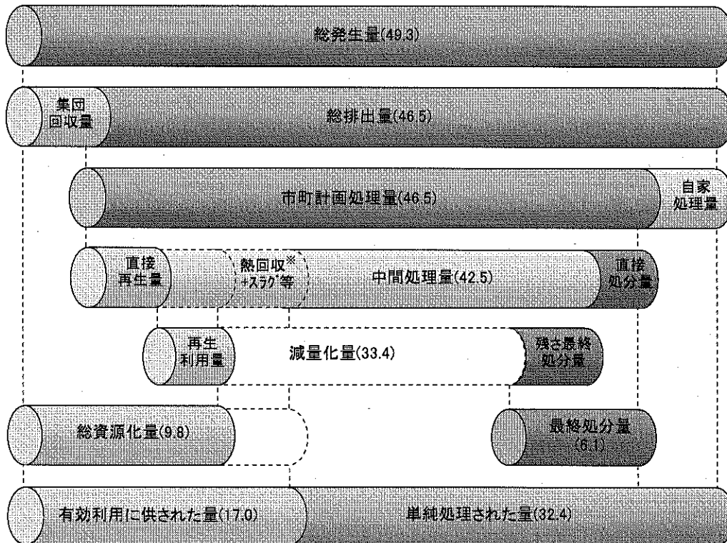
図 一般廃棄物の処理の概念図(平成19年度、万t/年)
