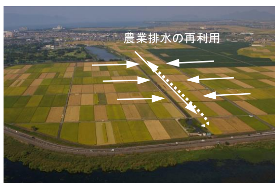
循環かんがい施設の例(木浜地区)
