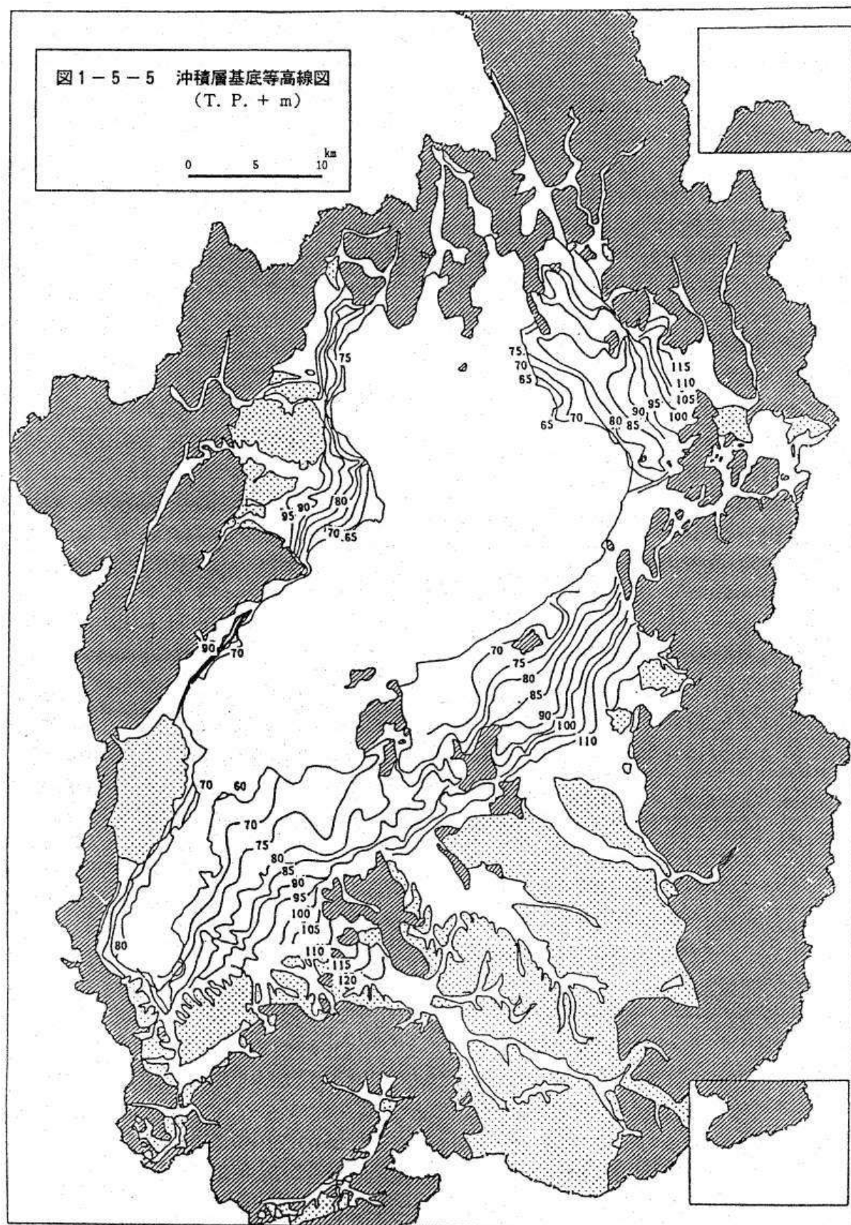
図1-5-5 沖積層基底等高線図
