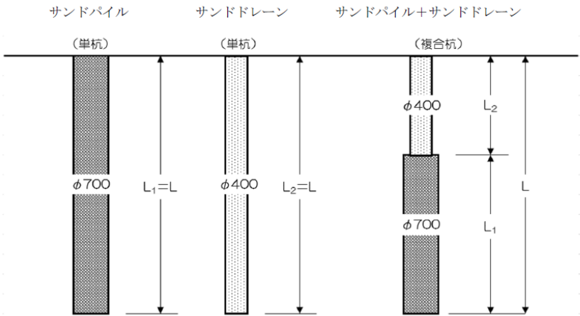
図 6－2 施工図
