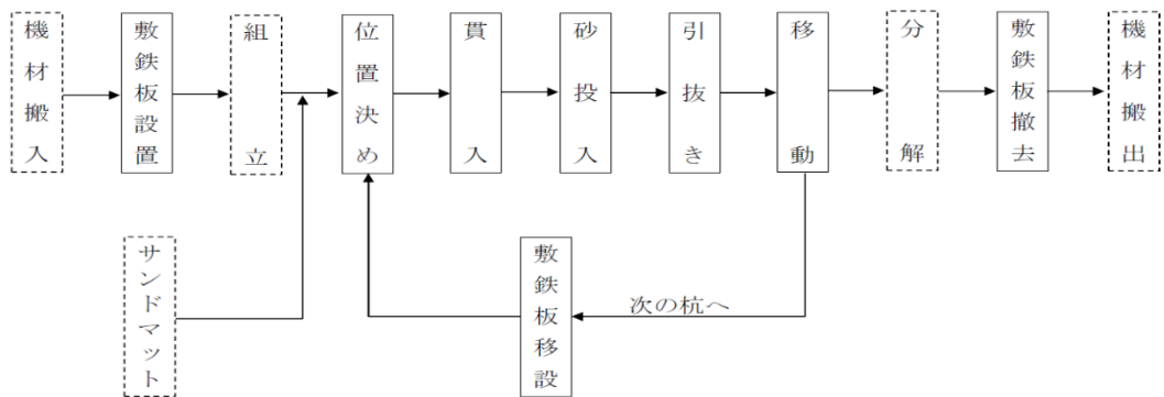
図 6－1 施工フロー
